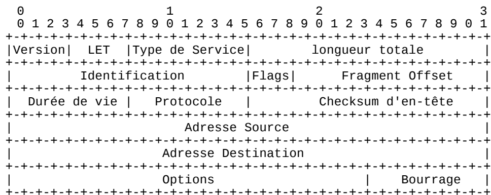
Exemple d'en-tête de Datagramme Internet Figure 4.
