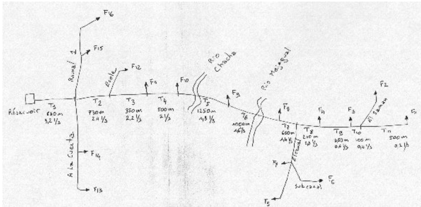
Schéma d'ensemble adduction La Romana.
