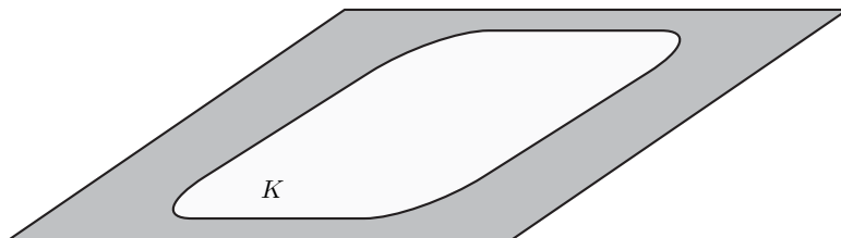
FIGURE 2. Voisinage de \infty
