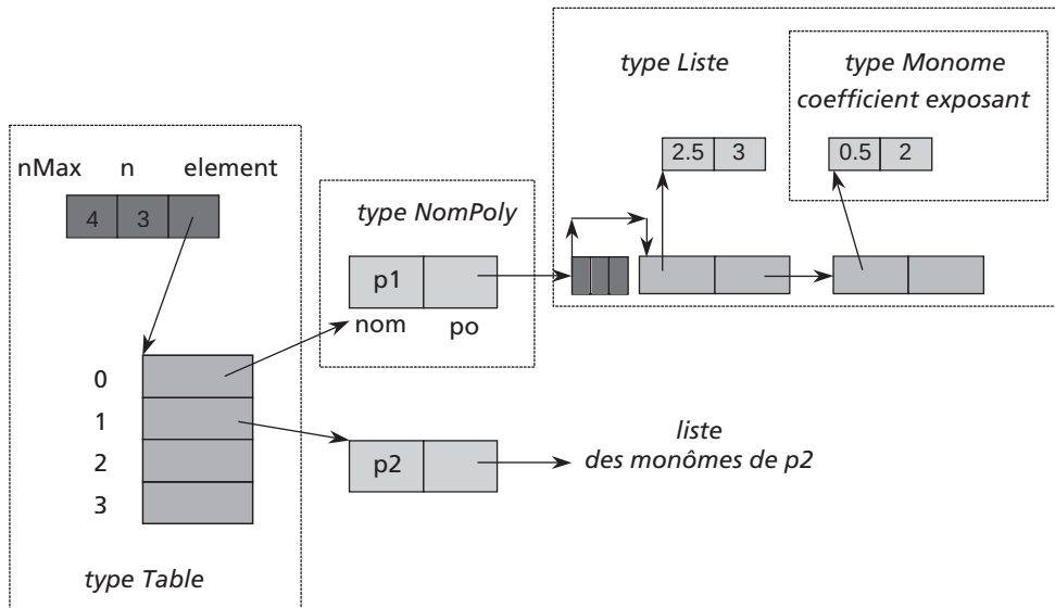
Figure 121 Détails de l'implémentation de la table.
