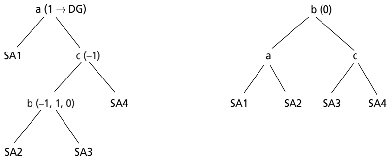
Figure 99 Principe de la réorganisation DG.
