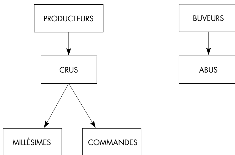
Figure IV.17 : Exemple de base hiérarchique
