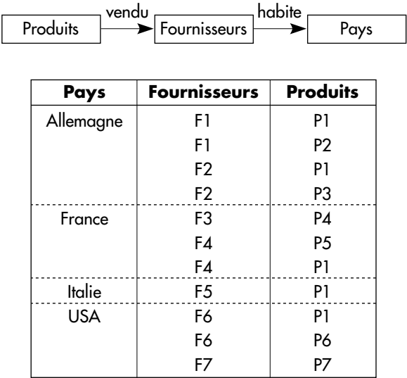
Figure XIV.4 : Exemple d'index de chemin simple
