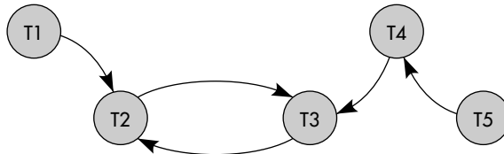
Figure XVI.15 : Transactions en situation de verrou mortel
