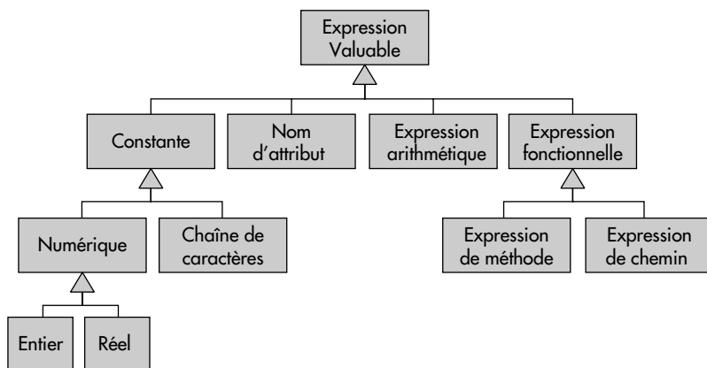
Figure XI.19 : Différents types d'expressions valuables
