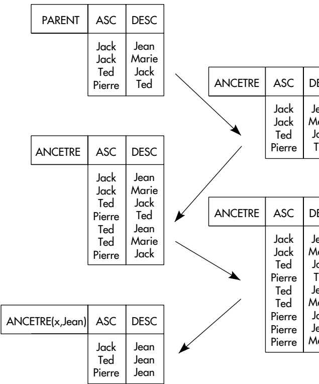
Figure XV.24 : Évaluation naïve des ancêtres de Jean
