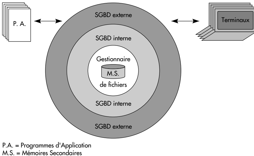
Figure I.1 : Première vue d'un SGBD
