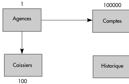
Figure XVI.1 : Schéma de la base TPC A
