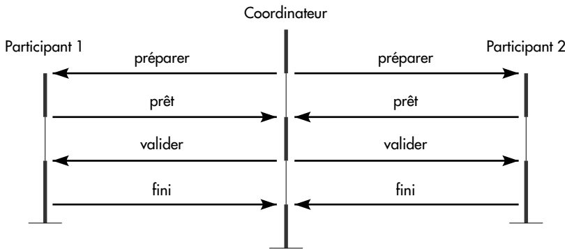
Figure XVI.37 : Validation en deux étapes avec succès
