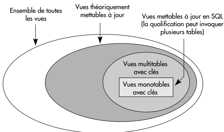
Figure IX.4 : Classification des vues selon les possibilités de mise à jour
