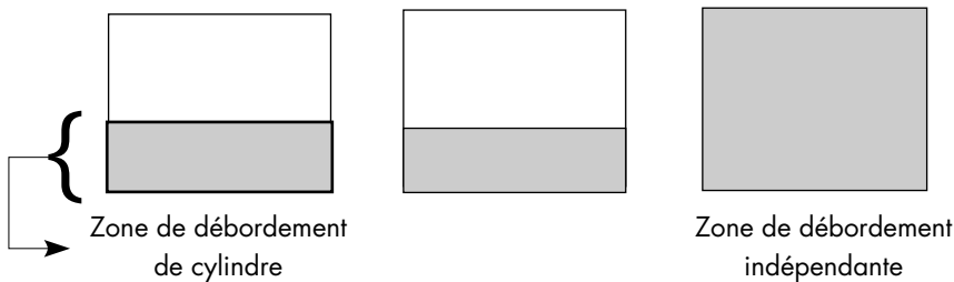
Figure III.22 : Zones de débordement d'un fichier ISAM.
