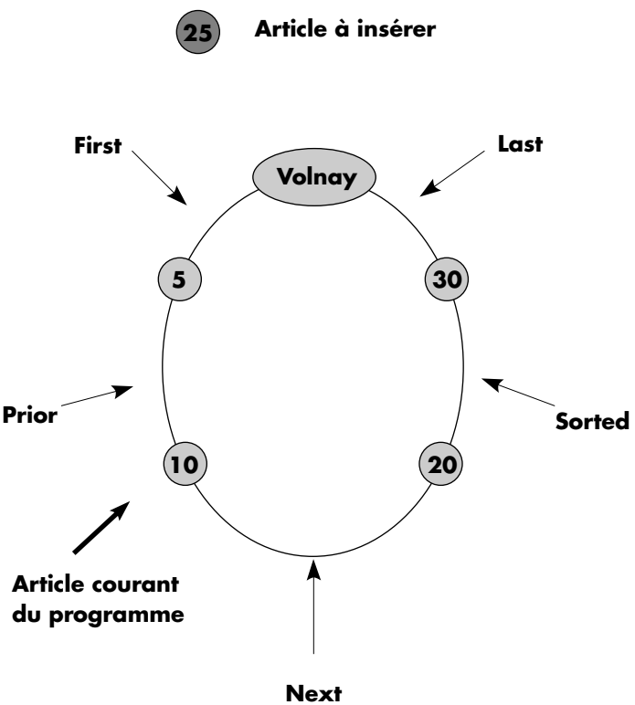
Figure IV.6 : Possibilités d'insertion dans une occurrence de lien
