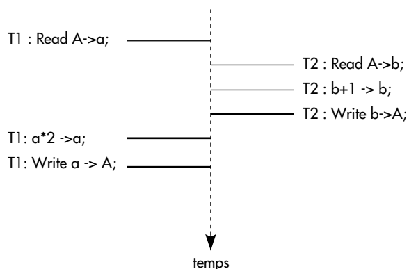
Figure XVI.3 : Exemple de perte de mise à jour
