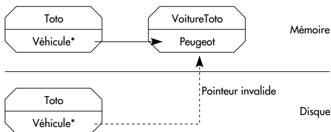
Figure XI.16 : Nécessité de mettre à jour les pointeurs en mémoire
