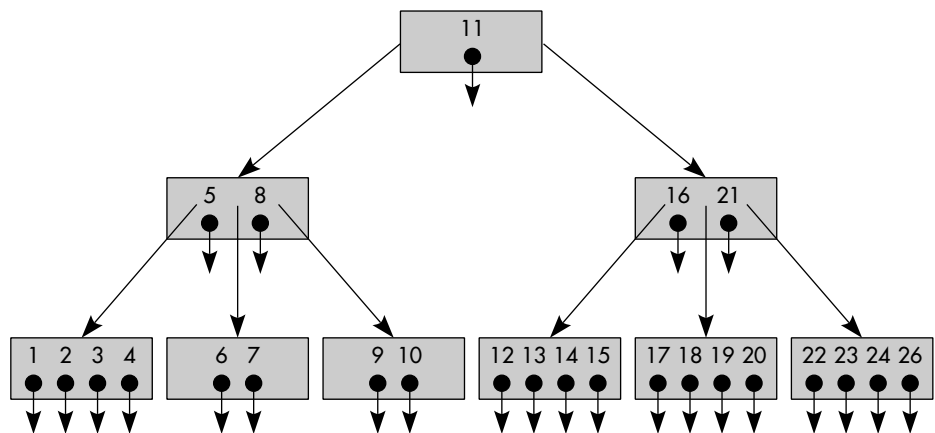
Figure III.17 : Exemple d'index sous forme d'arbre B
