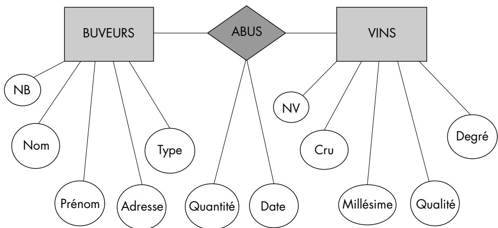
Figure VI.6 : Diagramme entité-association de la base DEGUSTATION
