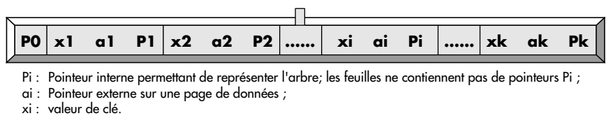
Figure III.16 : Structure d'un nœud d'un arbre B
