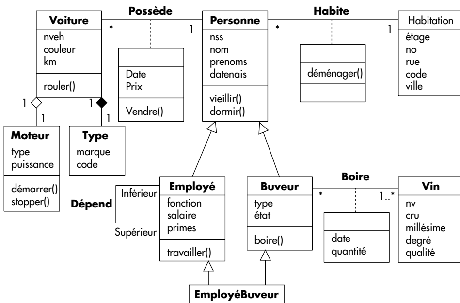
Figure XVII.12 : Exemple de schéma intégré UML
