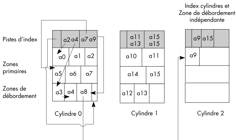
Figure III.24 : Vue d’ensemble d’un fichier ISAM (Les pointeurs issus du cylindre 1 ne sont pas représentés.)
