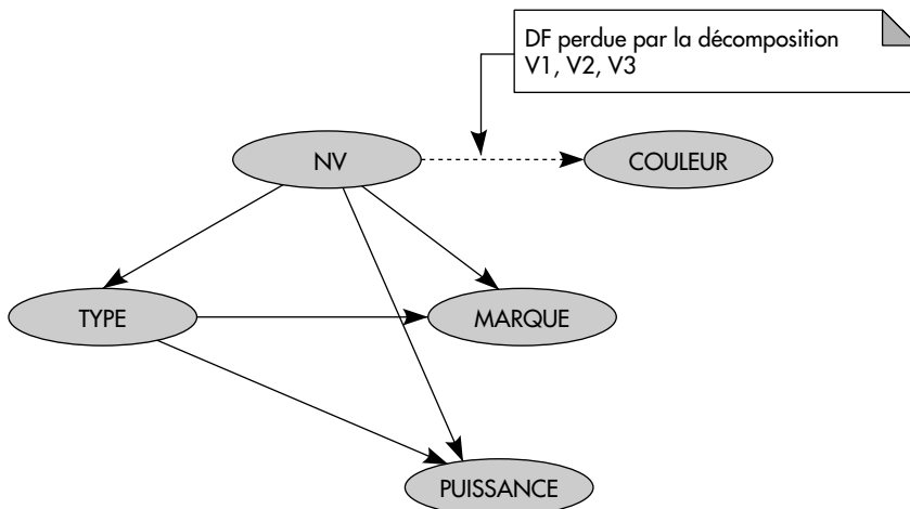
Figure XVII.28 : DF perdue par la décomposition \{V_1, V_2, V_3\}
