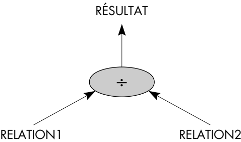
Figure VI.22 : Représentation graphique de la division
