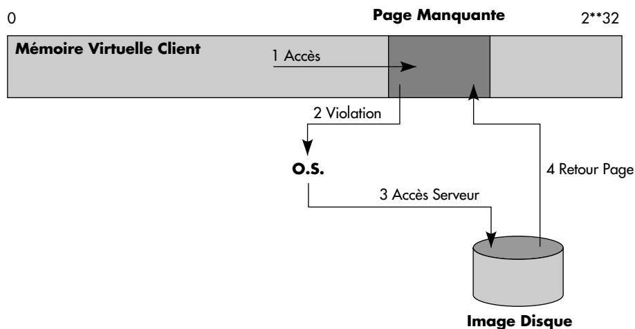
Figure XI.18 : La technique de mémoire virtuelle
