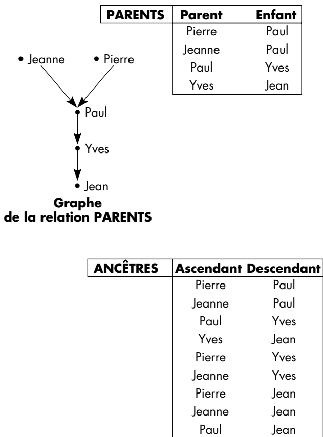
Figure VI.27 : Exemple de fermeture transitive
