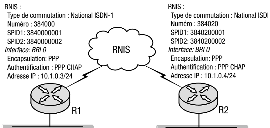
Listing 1.14. Configuration du routeur R1.
