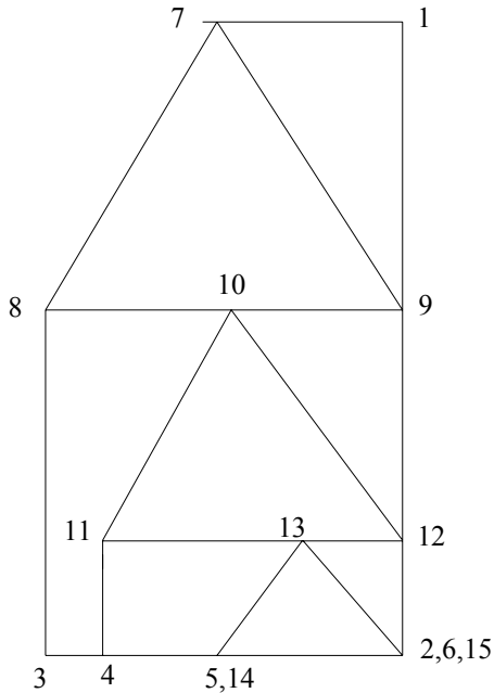
Diagramme des forces
