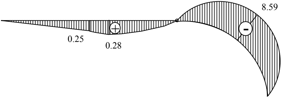
Diagramme du moment fléchissant M
