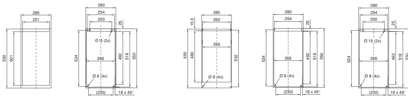
Découpe de montage, climatiseur partiellement intégré
