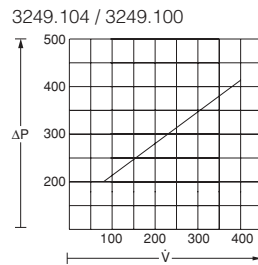
Diagrammes de résistance hydraulique Référence SK
