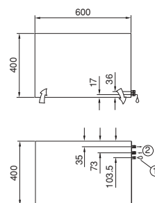
① = Evacuation de l'eau de condensation 1/2" ② = Connexion d'eau de refroidissement 1/2"
