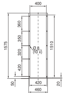
Découpe de montage, climatiseur intégré
