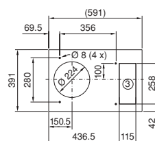
③ = Sortie d'air
