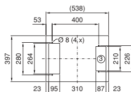
③ = Sortie d'air
