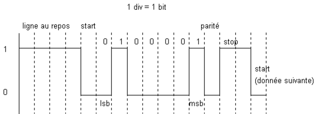
Illustration 6: Transmission série de l'octet 42 (caractère 'B')
