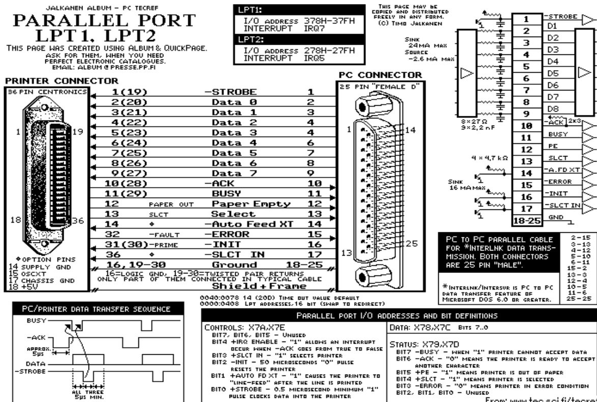
Illustration 3: Brochage de l'interface parallèle d'un PC (DB25 et Centronics)
