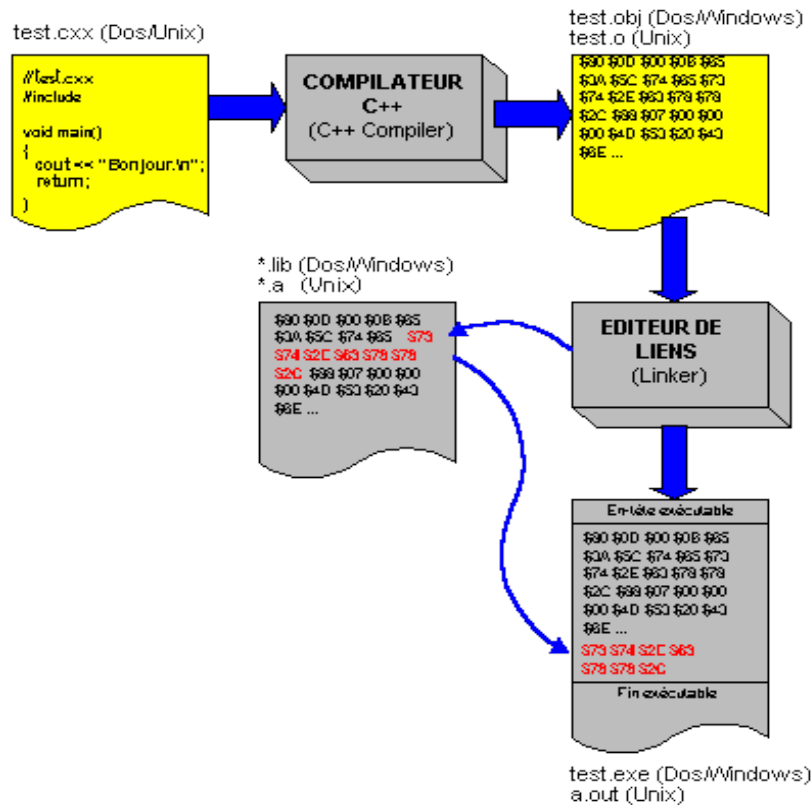
Illustration 1: Production d'un code exécutable
