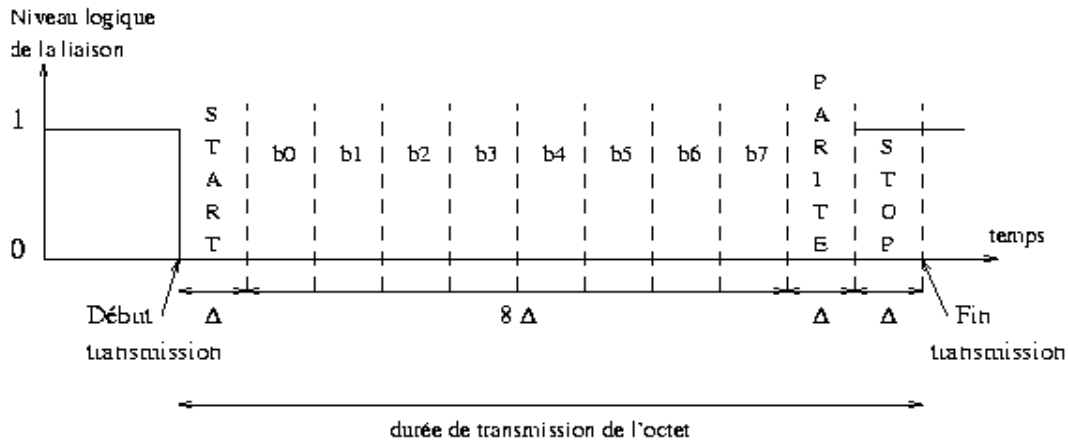
Illustration 5: Transmission d'un octet b_7 b_6 b_5 b_4 b_3 b_2 b_1 b_0 en série
