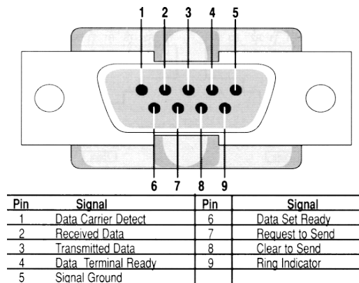
Illustration 8: Connecteur DB9
