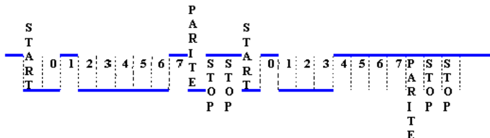
Illustration 7: Transmission de 2 octets avec une parité paire
