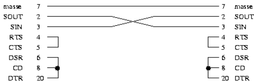
Illustration 10: Câble NULL-MODEM simplifié
