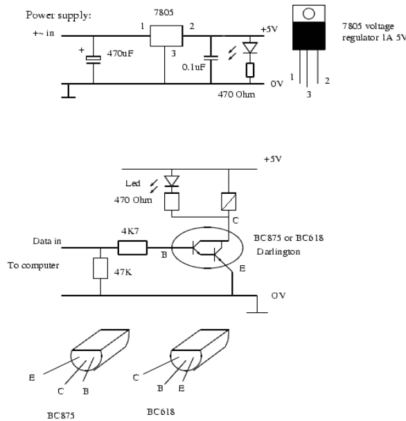
Illustration 4: Schéma de pilotage de relais depuis un port IEEE 1284
