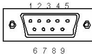
Connecteur mâle à 9 broches
