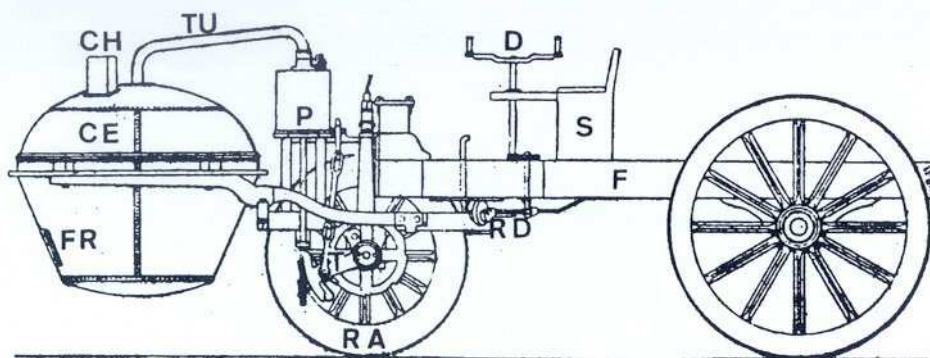
Croquis détaillé du fardier et de sa machine à vapeur (archives S.I.A.)
