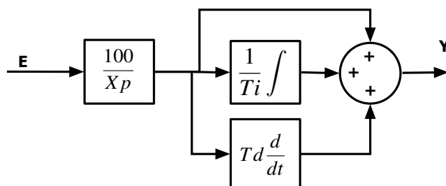
Structure mixte
