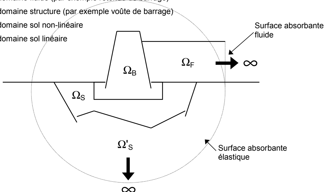
Figure 1.1-a : Domaine pour l'interaction sol-fluide-structure
