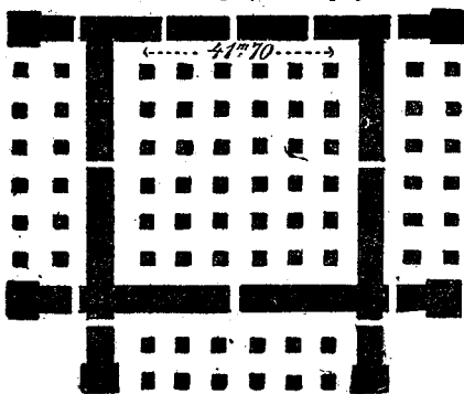
Galerie aux colonnes. (Palais royal de Persépolis.)
