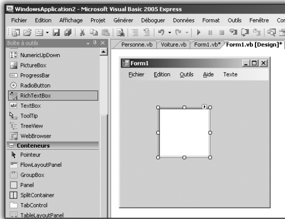
Figure 6.5 : Ajout d'une RichTextBox
