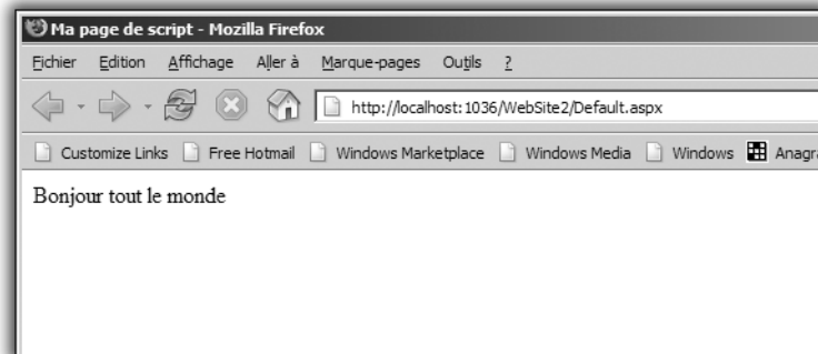
Figure 11.6 : Les fonctions
