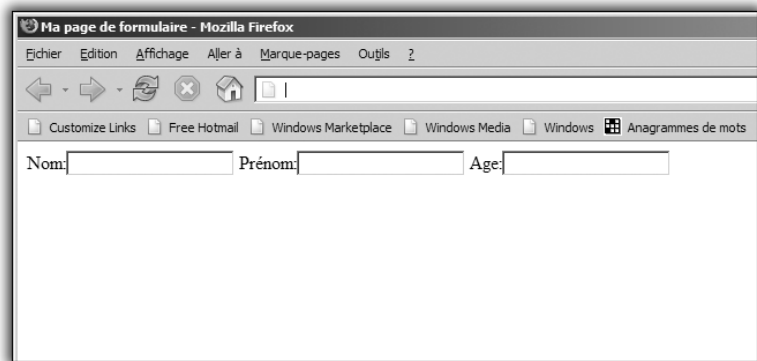
Figure 12.2 : Le formulaire
