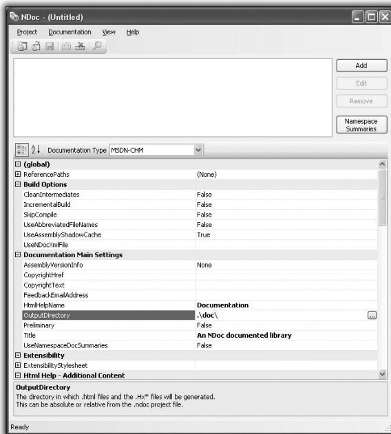
Figure 9.64 : Lancement de NDoc
