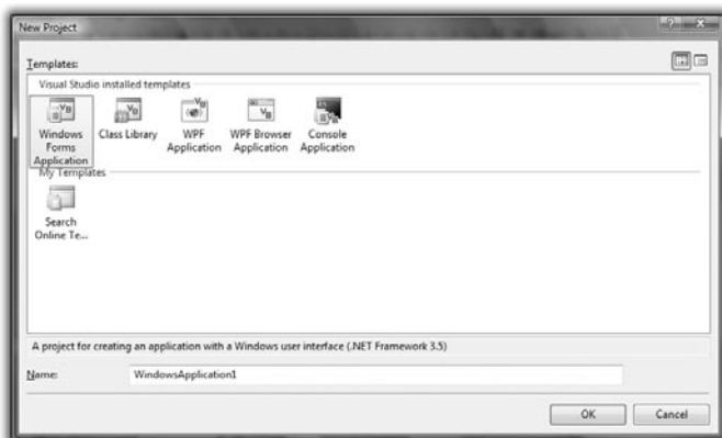
Figure 1.2 : Choix d'application
