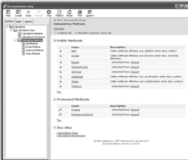
Figure 9.72 : Documentation finale
