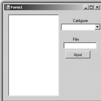
Figure 5.18 : Bibliothèque améliorée
