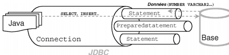
Figure 9-4 Connexion et états
