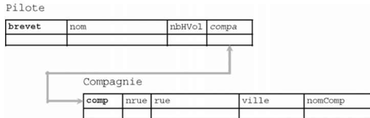
Figure 1-2 Deux tables à créer
