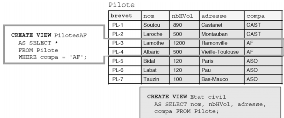
Figure 5-19 Deux vues d'une table
