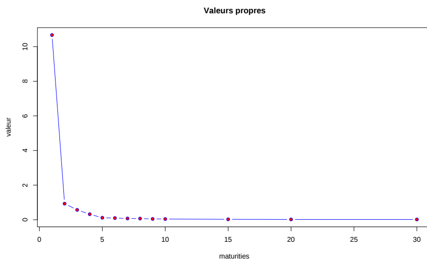
FIG. 6.3 – Valeurs propres
