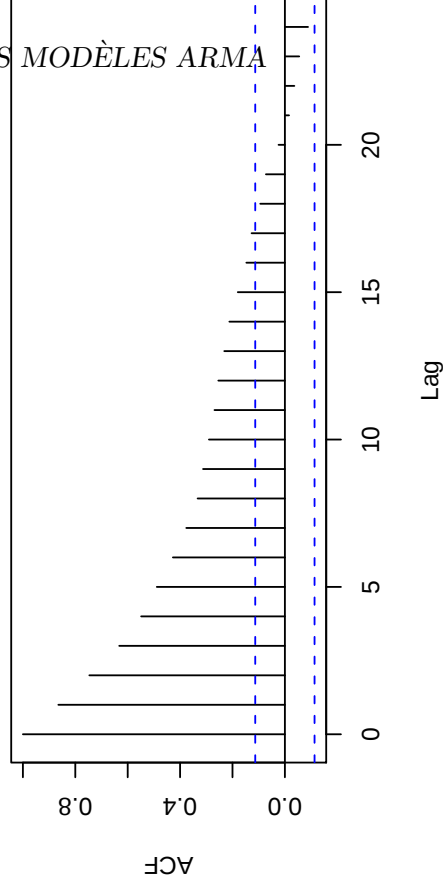
AR(1)
