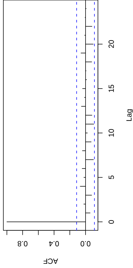
Bruit blanc
