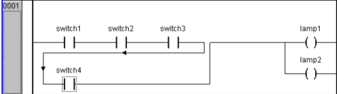
Exemple: Réseau avec mises en page
