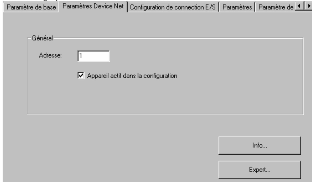
Boîte de dialogue pour Paramètres DeviceNet d'un Esclave DeviceNet
