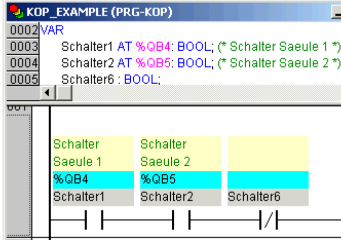
Exemple: Réseau avec affichage du commentaire des variables et de l'adresse de chaque contact
