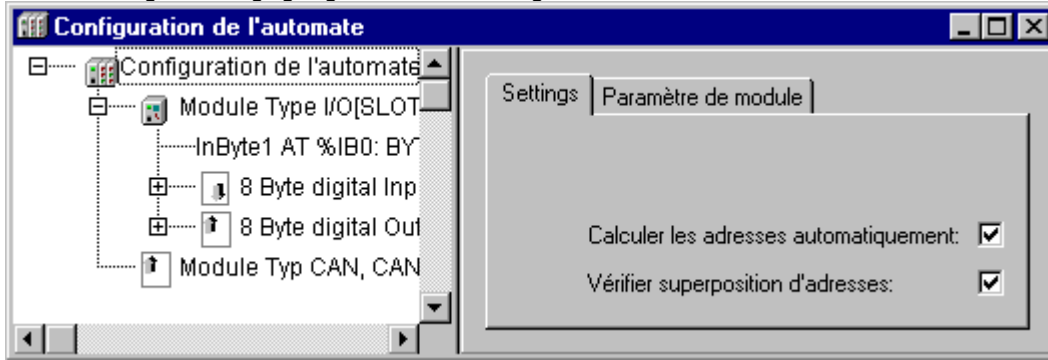
Boîte de dialogue des réglages généraux de la configuration d'automates
