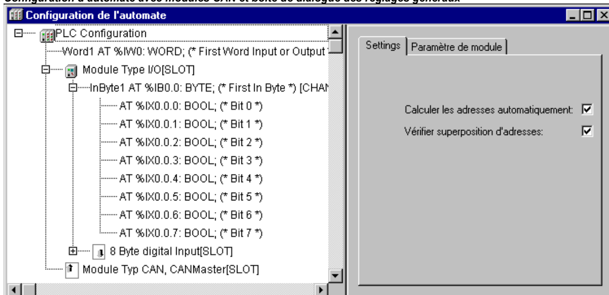
Configuration d'automate avec modules CAN et boîte de dialogue des réglages généraux
