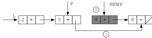
FIG. 2.2: Suppression d'un enregistrement d'une liste
