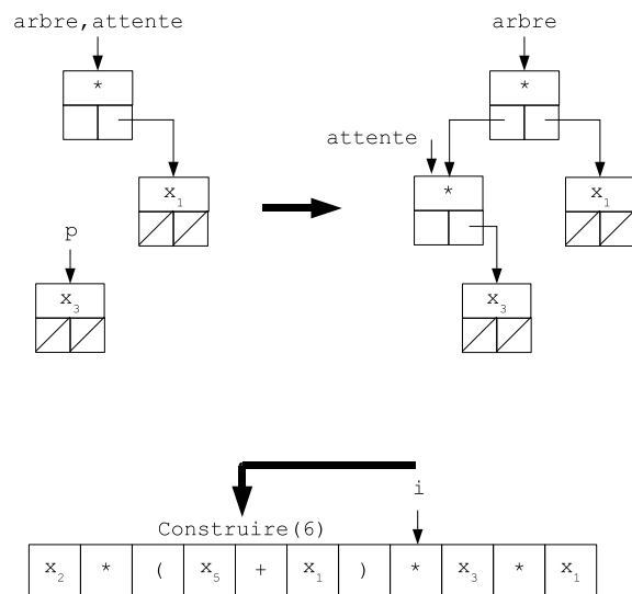
FIG. 4.15: Analyse d'une parenthèse fermante
