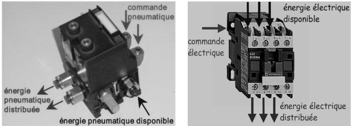
Figure 30: pré actionneurs
