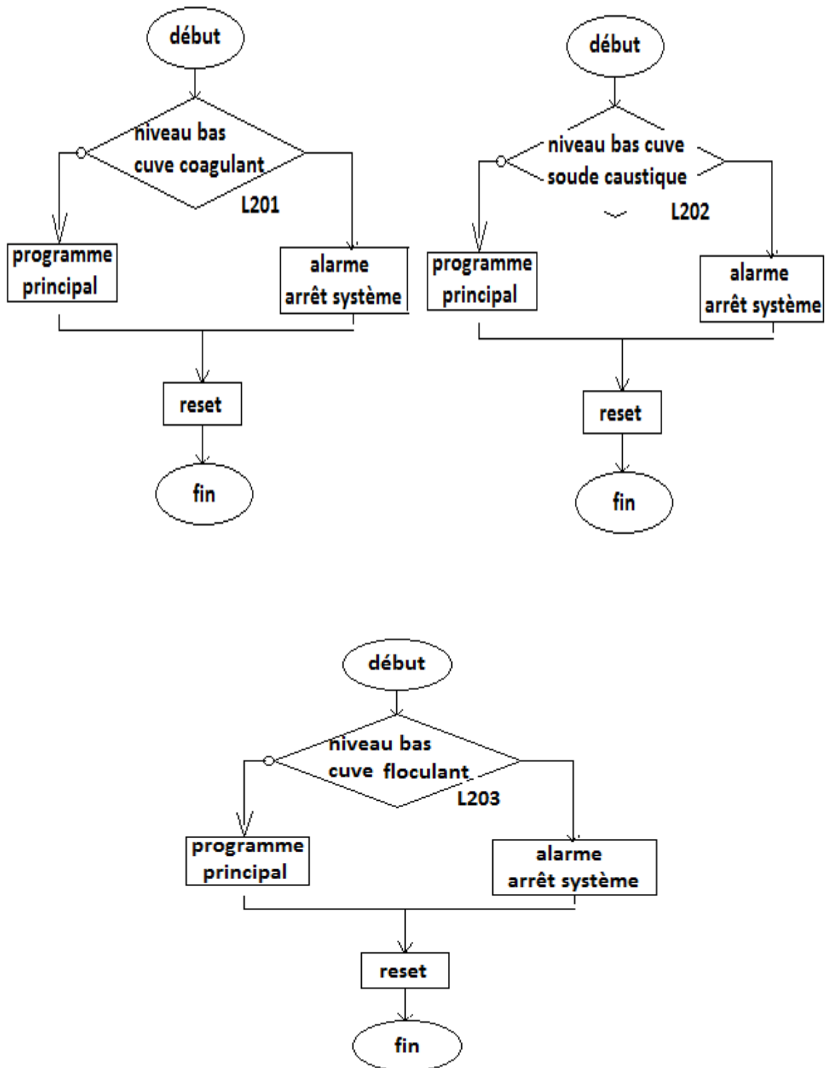
Figure 39: système d'injection de produits chimiques
