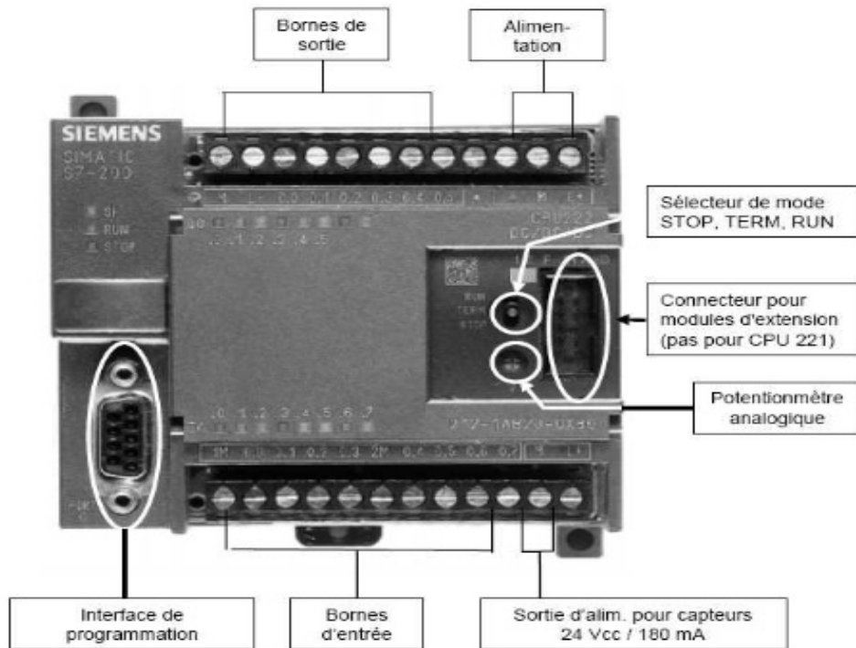
Figure 35: aspect extérieur d'un API S7_200
