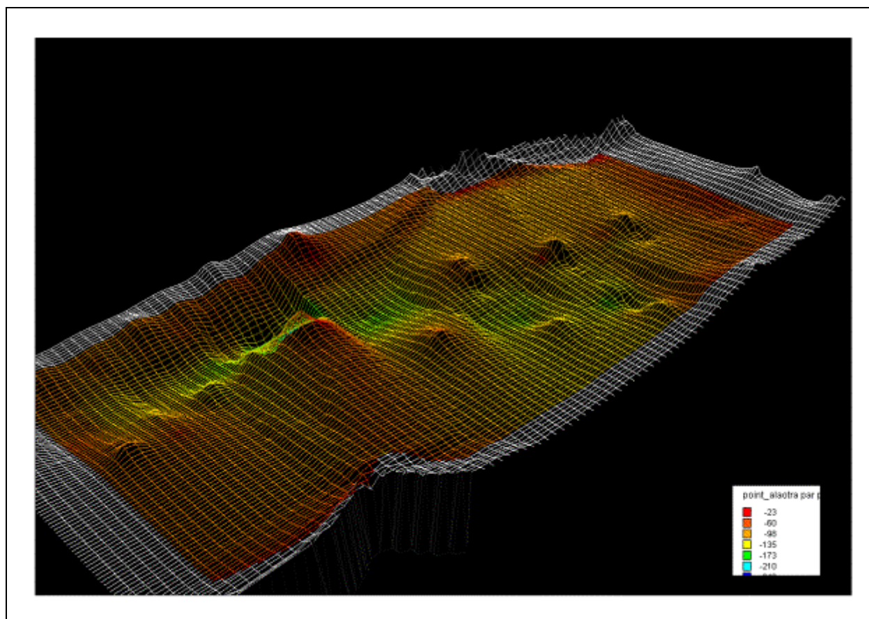
Figure 1 : Schéma montrant la visualisation du balayage de 100 m suivant la longueur et de 10m suivant la largeur (côté Est)
