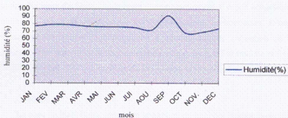
Figure 04. Humidité relative
