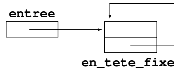
FIG. 3 – Maillon fixe en tête d'une liste chaînée
