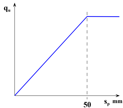
Fig. 18.4b Loi de mobilisation simplifiée de la résistance de pointe q_u
