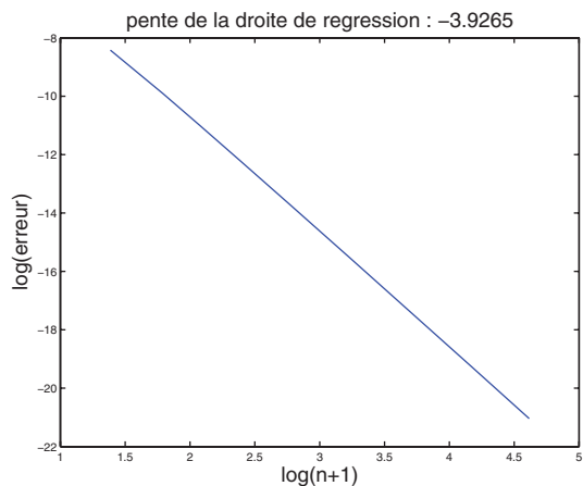
erreurs pour les fonctions f_1 et f_3
