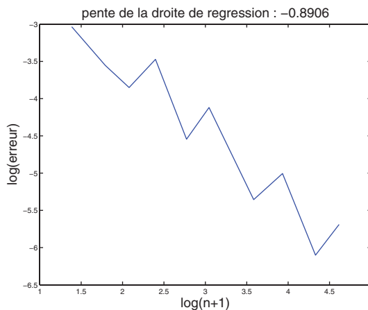
erreurs pour les fonctions f_1 et f_3
