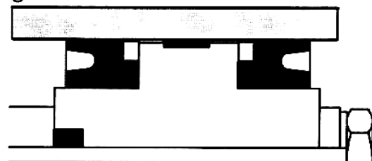
Joints à double lèvre soutenus avec segment
