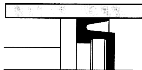
Manchette à double lèvre enclavée
