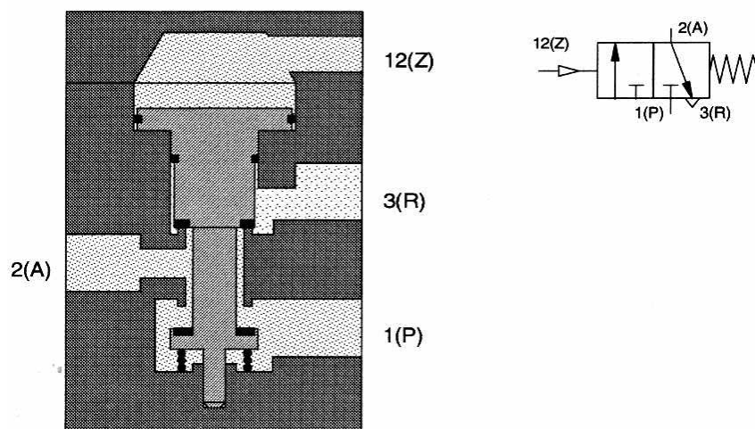
Distributeur 3/2 à commande pneumatique, fermé au repos, actionné b)
