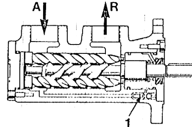
Pompe à vis.
