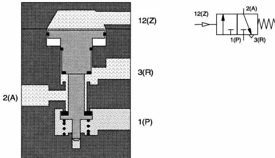
Distributeur 3/2 à commande pneumatique, fermé au repos, non actionné a)
