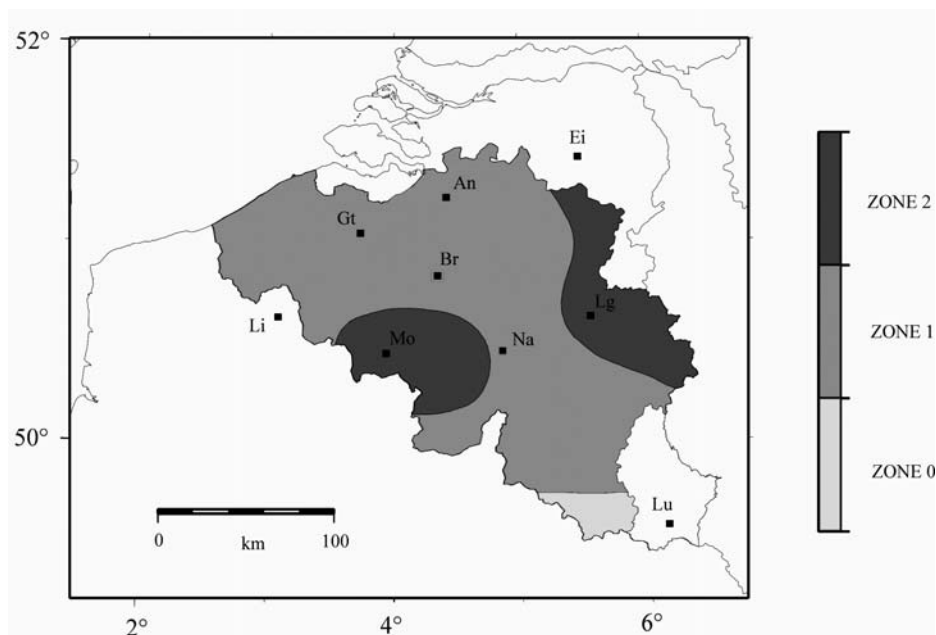
Figure 1.7. Carte de zonage sismique de la Belgique.
