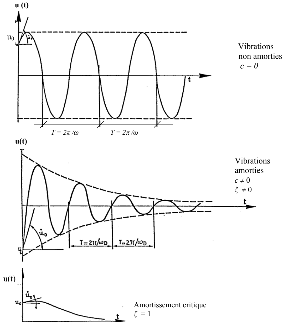
Figure 2.2. Types de vibrations libres ( p(t)=0 ) réalisées par écartement u_0 de la position d'équilibre.
