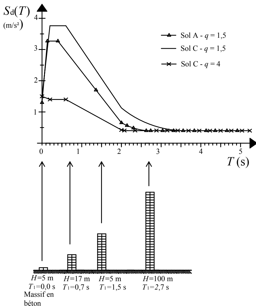
Figure 2.9. Exemples de spectre de calcul pour divers sites et coefficient de comportement, en regard de quelques structures caractérisées par leurs périodes T_1 (estimée par la relation T_1 = Ct H^{3/4} du Tableau 2.3).
