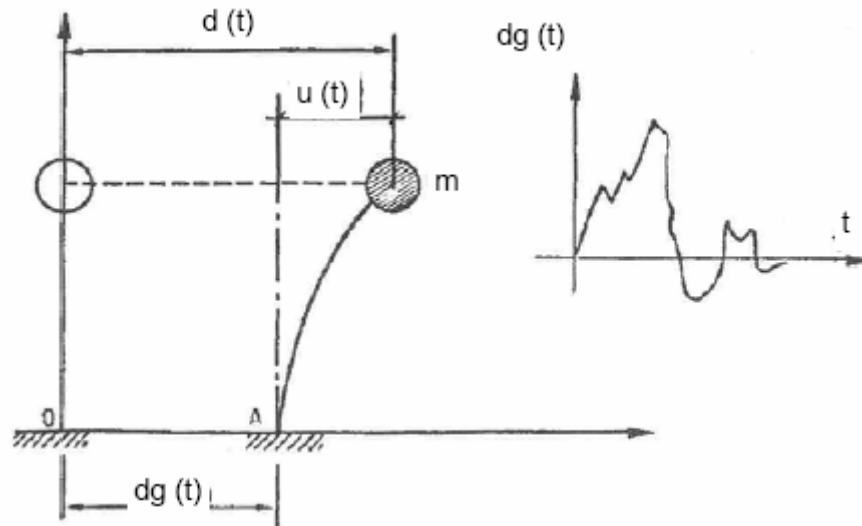
Figure 2.4. Excitation d'une structure par déplacement horizontal de son appui.
