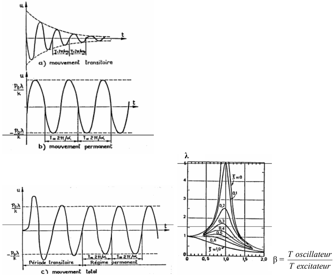
Figure 2.3. Oscillations forcées harmoniques et coefficient d'amplification \lambda du déplacement.
