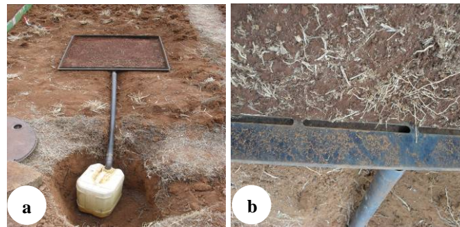
Cliché 3: Micro-lots d'érosion : (a) cadre mis en place avec ses équipements – (b) Fentes sur la face en aval du cadre _ Source : Laingo, 2010
