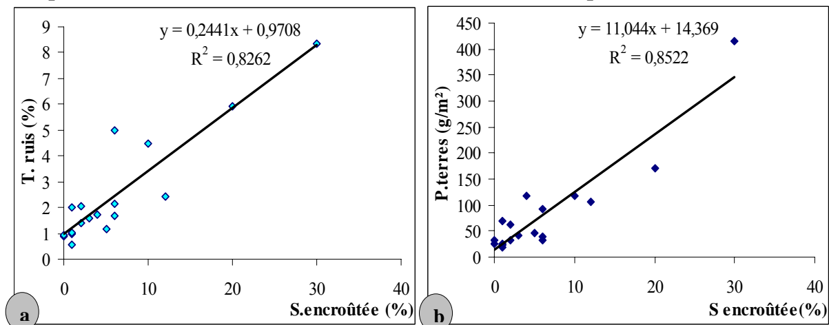
Figure 13 : Relation entre le pourcentage de surface encroûtée après saison pluvieuse et (a) le taux de ruissellement - (b) de l'érosion durant la saison pluvieuse.
