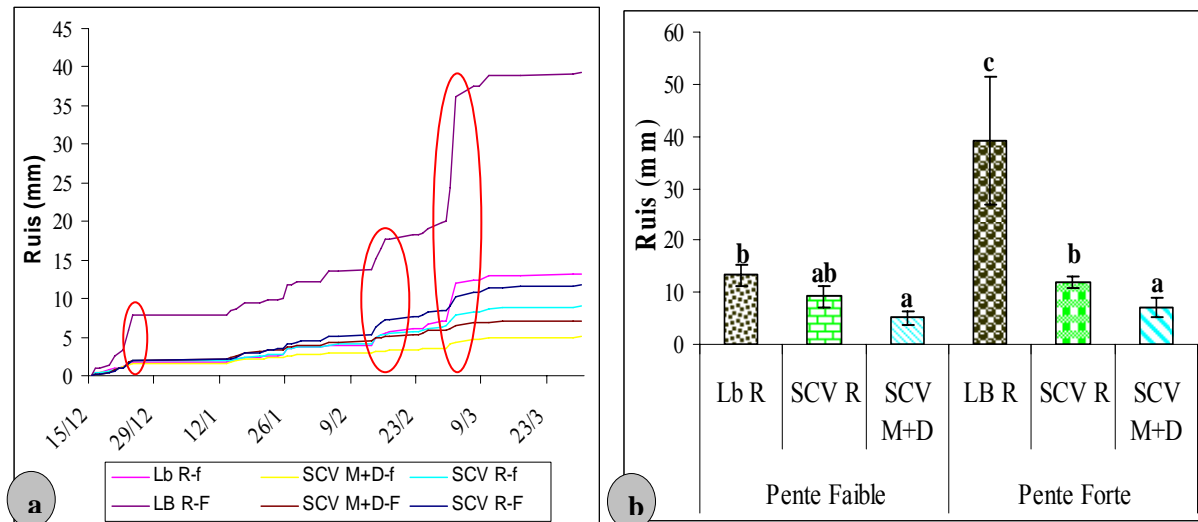
Figure 8 : Ruissellement durant la campagne pluvieuse 2010-2011 : (a) Dynamique de ruissellement en fonction de la date des pluies – (b) Cumul de ruissellement en fonction du traitement et de la pente
