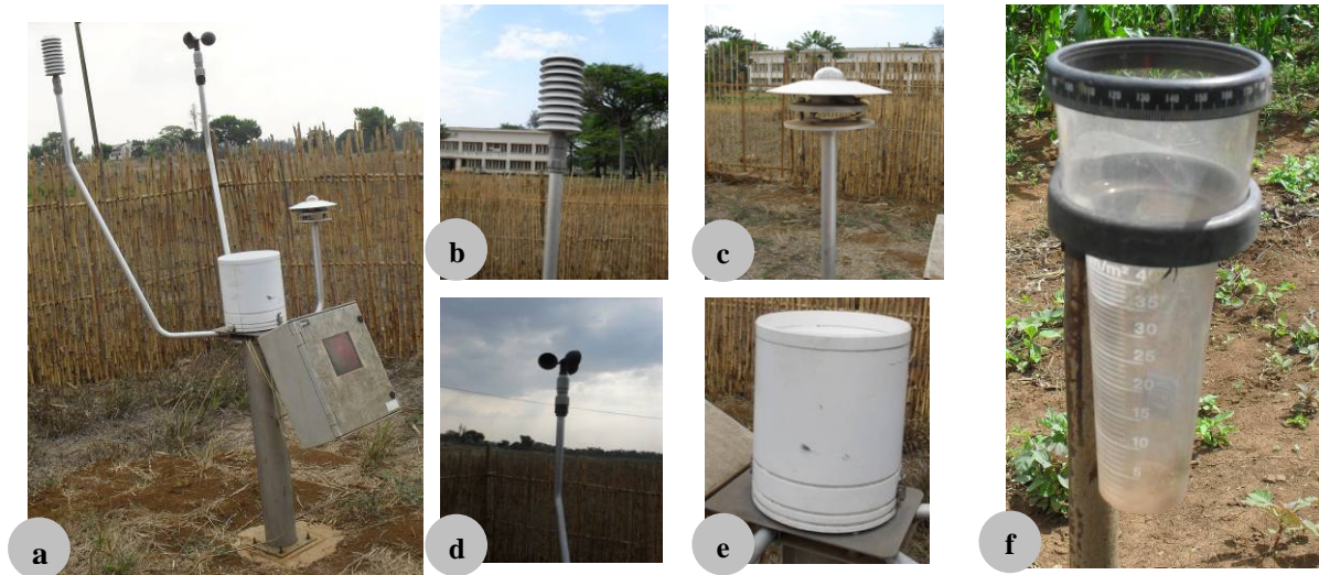
Cliché 2 : Station météorologique : (a) station automatique de CIMEL : (b) Capteur de température et d'humidité dans un Mini Abri – (c) Pyranomètre – (d) Anémomètre – (e) Pluviomètre
