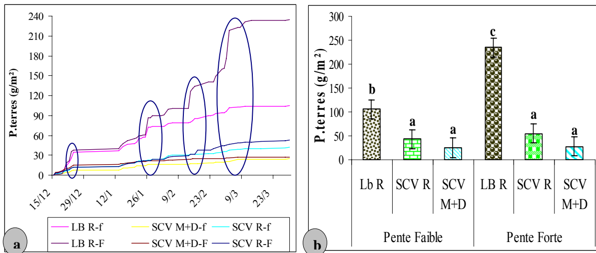
Figure 9: Pertes en terre durant la saison pluvieuse 2010-2011 : (a) Dynamique des pertes en terres en fonction de la date des pluies – (b) Pertes en terres en fonction des traitements et des pentes
