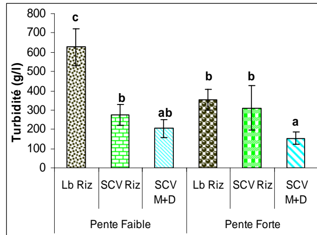
Figure 10 : Turbidité en fonction du traitement sur des pentes différentes
