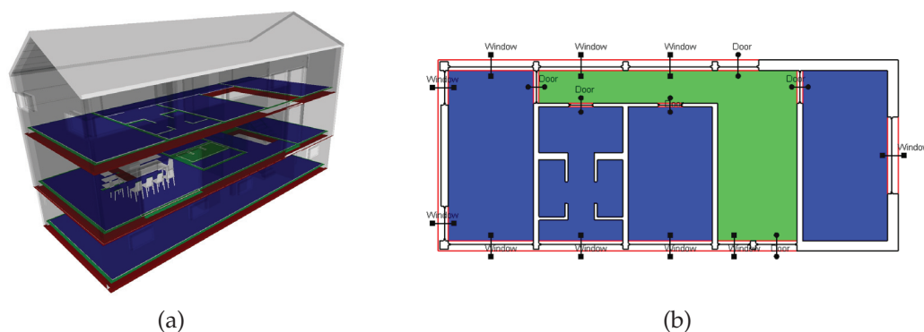
FIGURE 26 – Images issues de [157]. (a) Modèle 3D d'un immeuble de trois étages. Les surfaces rouges constituent des plafonds et les bleues représentent les planchers. (b) Graphe de connectivité représentant les pièces (bleues), les couloirs (en vert), les parois et ouvertures.
