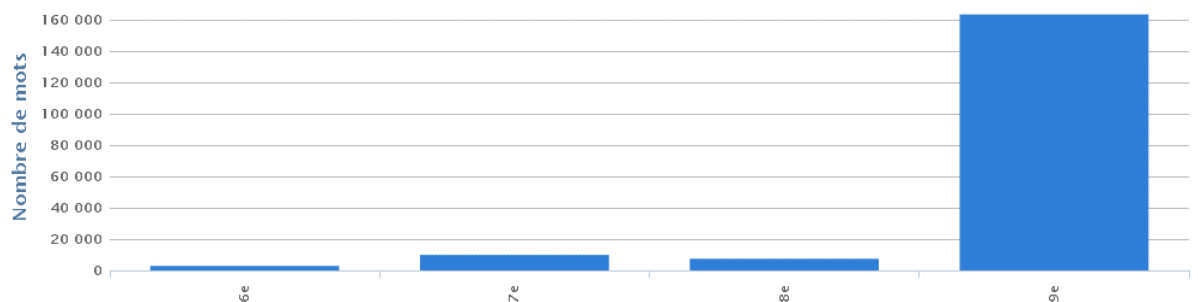
Figure 9 : Dimension du corpus CBMA par siècle (6 e –9 e )
