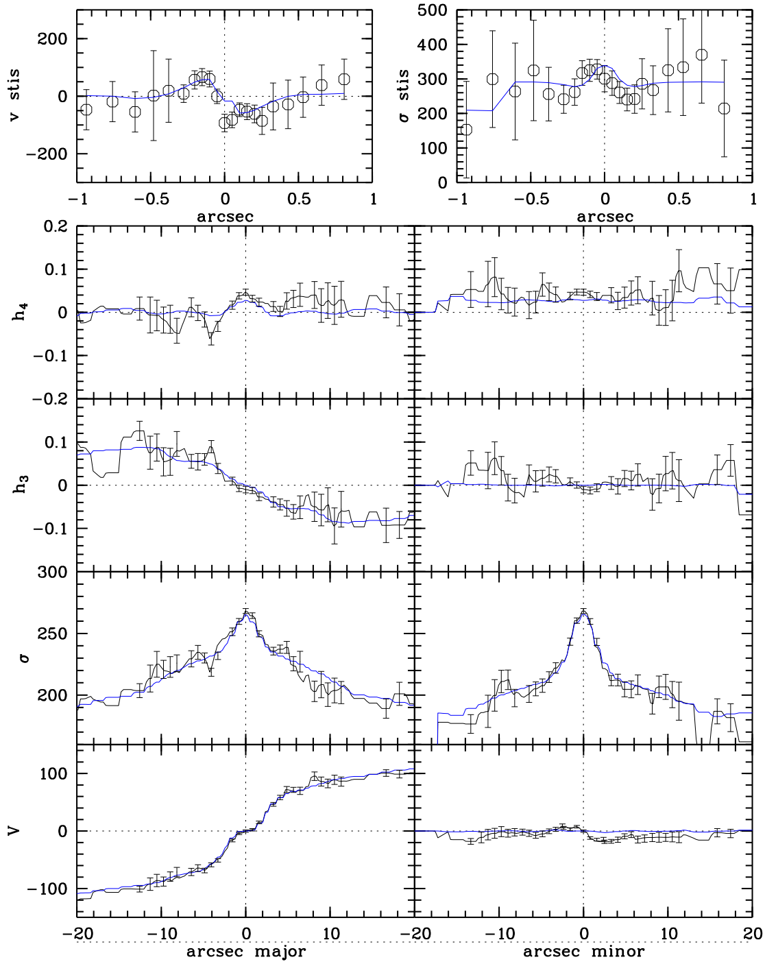
FIG. II.20 – Coupe des données saupon de NGC 4621 le long des axes principaux de la galaxie. La courbe pleine correspond au modèle à trois IDM de Schwarzschild.
