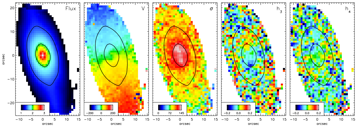
FIG. III.15 – Champs des paramètres cinématiques de NGC 7332 avec sapron (Figure tirée de la thèse de Falcón-Barroso (2002)).
