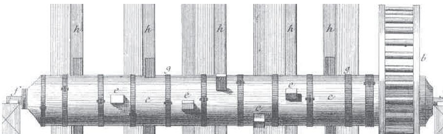
Figure 35 : Arbre de hérisson.
