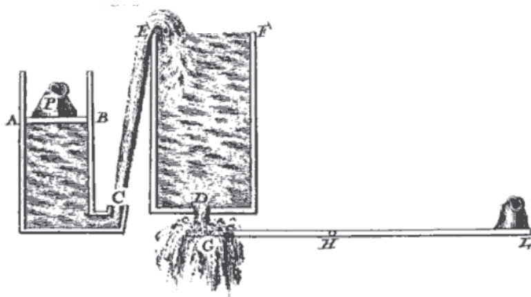
Figure 48 : Pompe alimentant un réservoir ouvert en D, permettant au fluide de frapper la pale HG
