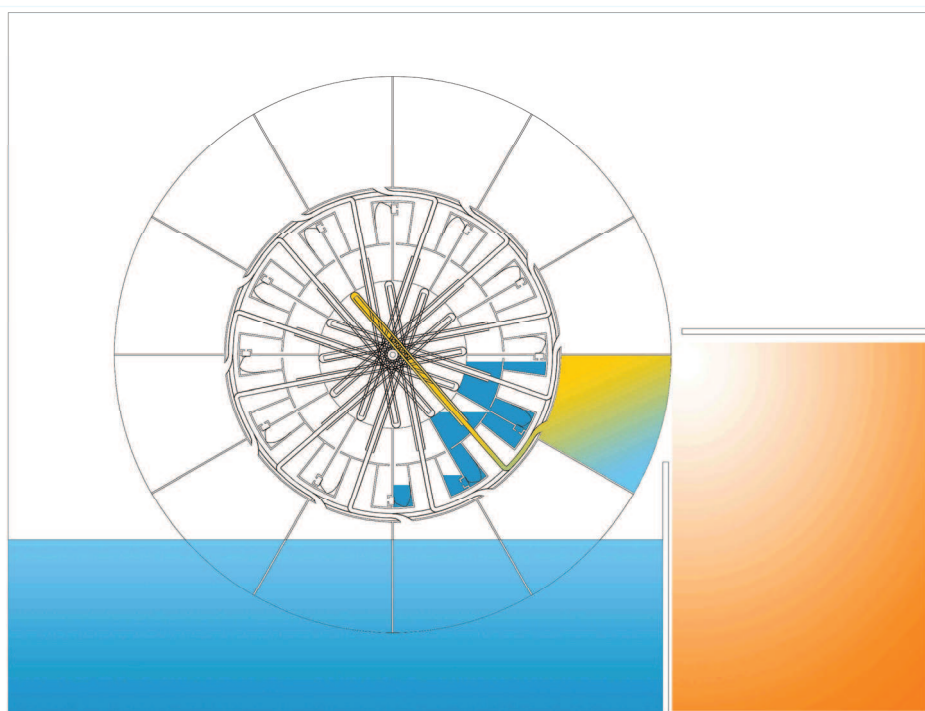
Figure 19 : Version réalisée informatiquement du moulin d'Amontons.
