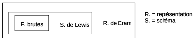
Figure 8 – Représentation de certains emboîtements des représentations moléculaires
