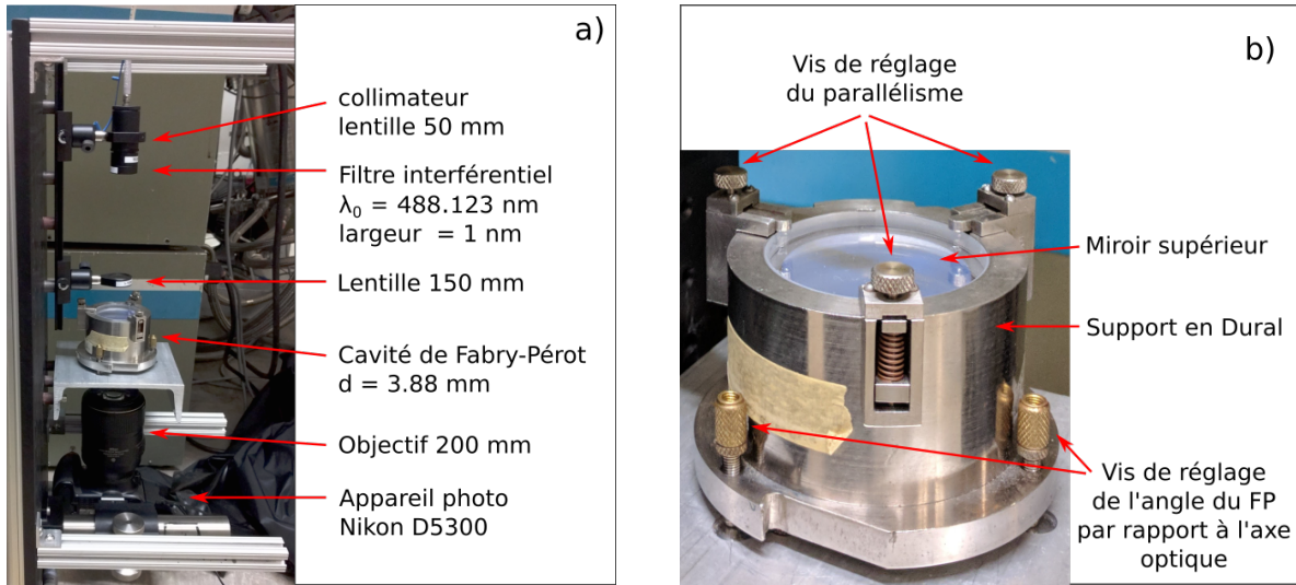
FIGURE 1.25 – a) Partie finale du dispositif d’interf rom trie Fabry-P rot, b) cellule de Fabry-P rot.
