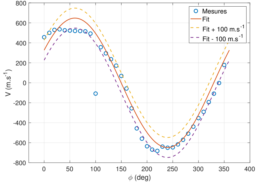
FIGURE 1.17 – Vitesse des ions mesurée par sonde de Mach en fonction de l’angle de la sonde avec la direction azimuthale et fit de cette courbe d’après l’équation 1.21. Le fit est également tracé associé à l’erreur expérimentale typique de \pm 100 \text{ m.s}^{-1} .
