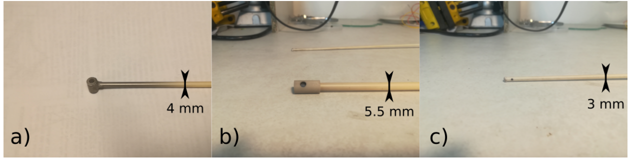
FIGURE 1.14 – Trois designs successifs de sondes de Mach : a) design final avec une tête de sonde en "T" en nitrure de bore et des collecteurs plats, b) design avec un chapeau en alumine et des collecteurs plats et c) design en trou d'épingle, directement percé dans le corps de la sonde en alumine et avec un conducteur en fil de tantale.
