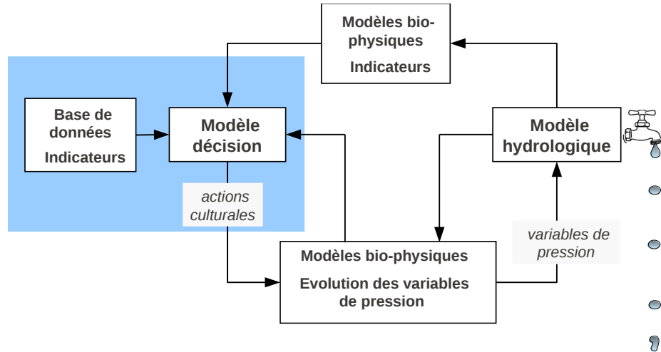
FIGURE 1.15 – La partie du modèle conceptuel traitée dans la partie I
