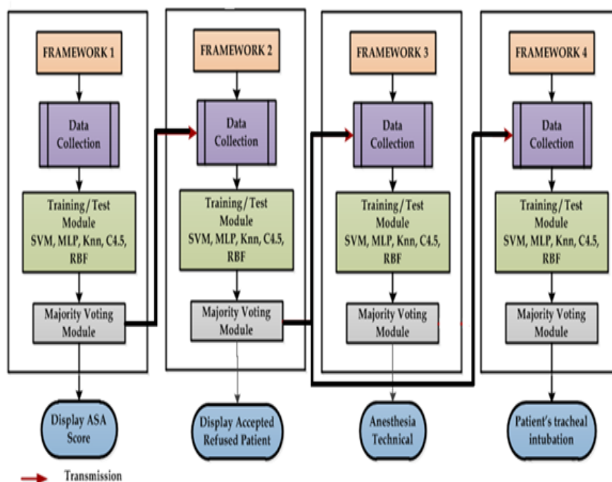
FIGURE 4.1 – Schéma bloc du prototype proposé
