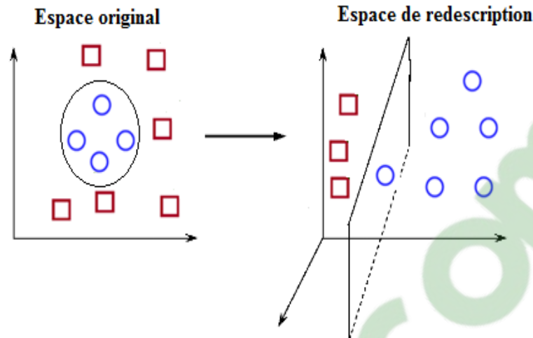
FIGURE 4.7 – Transformation d'espace
