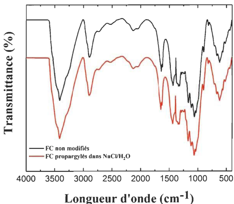
Figure 43 Spectres IR des FC non modifiés et FC propargylés dans le système \text{NaCl}/\text{H}_2\text{O}
