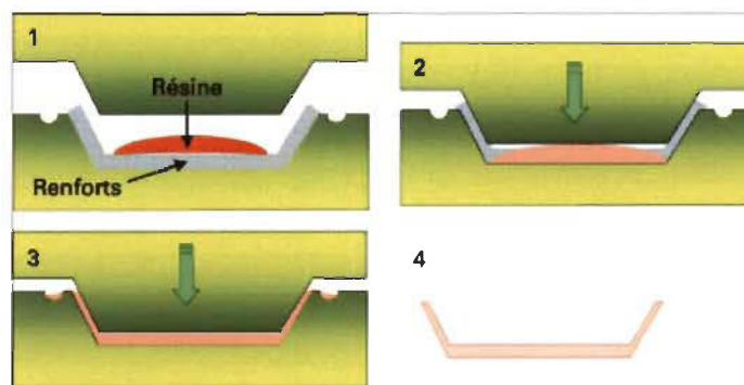
Figure 12 Schéma du procédé de moulage par compression
