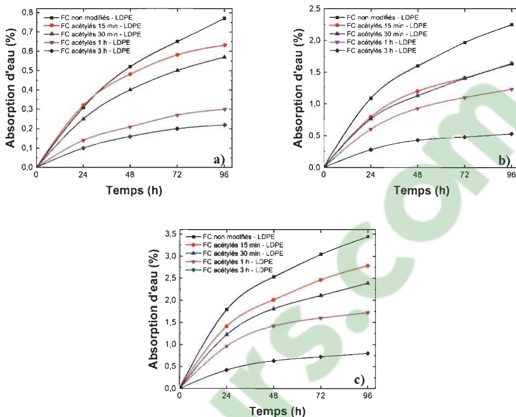
Figure 42 Absorption d'eau des composites en fonction du temps pour a) 10%, b) 20% et c) 30% de FC
