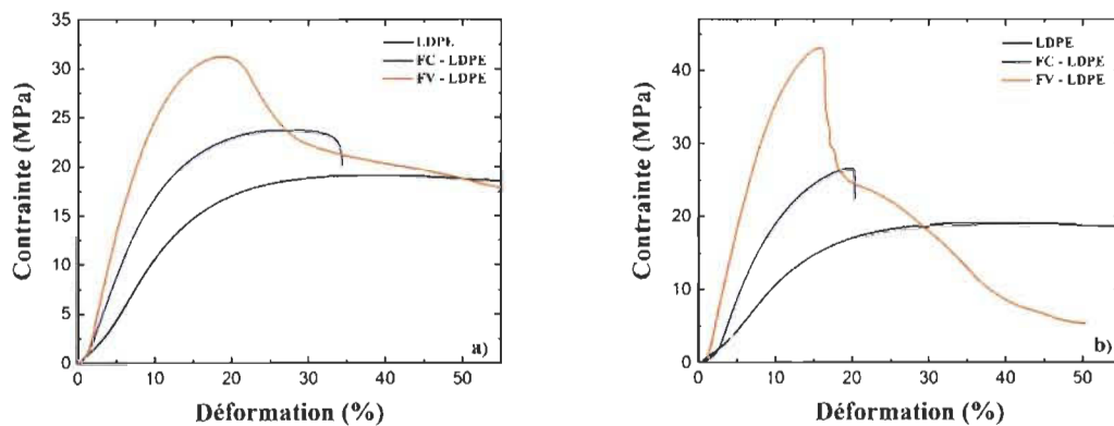
Figure 28 Courbes contrainte/déformation des composites FC-LDPE et FV-LDPE pour une teneur en renfort de : a) 10% et b) 20%
