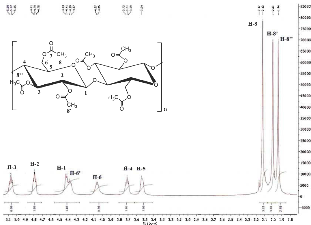
Figure 35 Spectre RMN ^1\text{H} des filaments de cellulose acétylés 72 h
