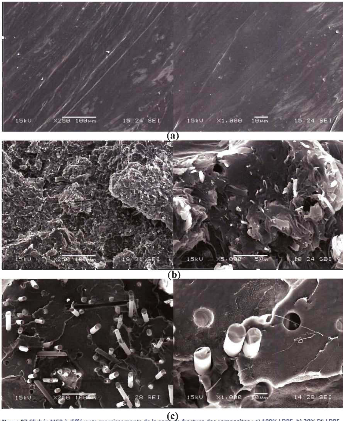
Figure 27 Clichés MEB à différents grossissements de la zone de fracture des composites : a) 100% LDPE, b) 20% FC-LDPE et c) 20% FV-LDPE
