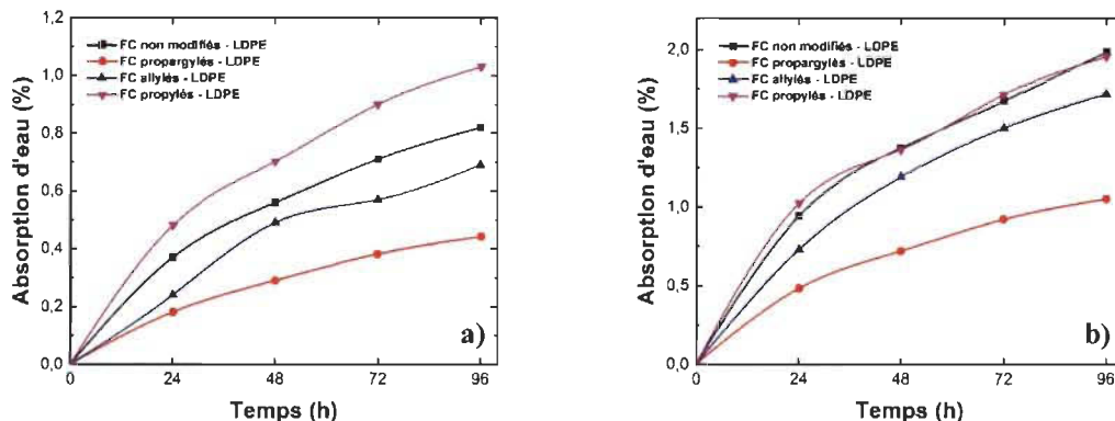
Figure 58 Absorption d'eau des composites en fonction du temps pour a) 10% et b) 20% de FC
