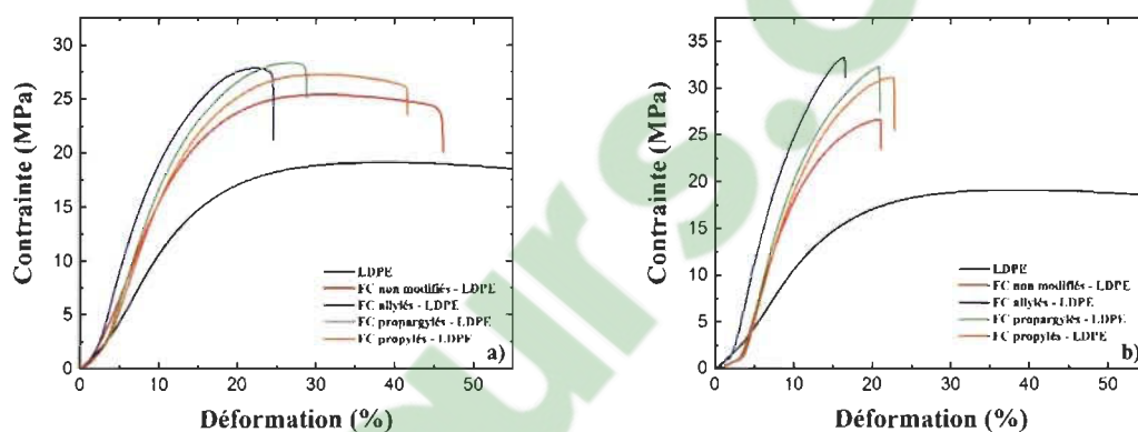
Figure 55 Courbes contrainte/déformation des composites à base de FC non modifiés et alkylés pour une teneur en filaments de : a) 10% et b) 20%
