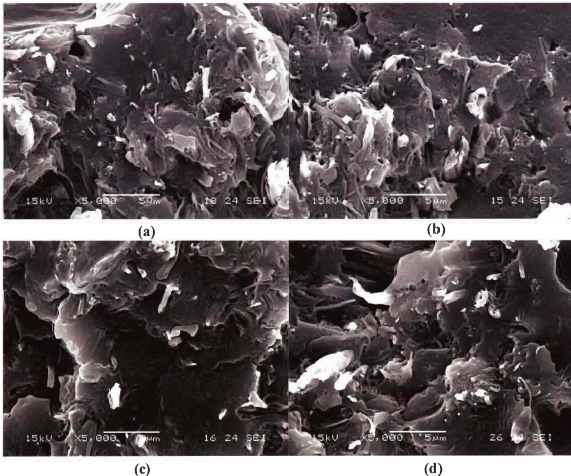
Figure 54 Observations MEB des zones de fracture des composites : a) 20% FC non modifiés + LDPE, b) 20% FC propargylés + LDPE, c) 20% FC allylés + LDPE et d) 20% FC propargylés + LDPE
