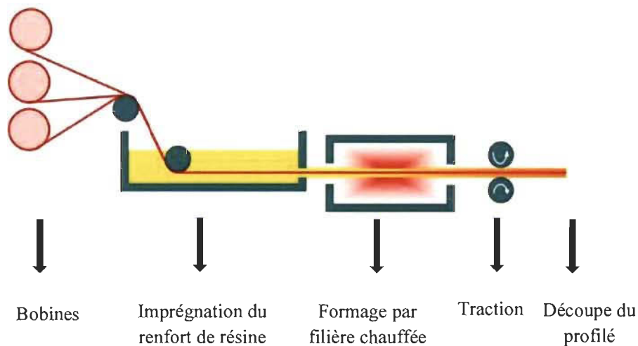
Figure 14 Schéma du procédé de pultrusion
