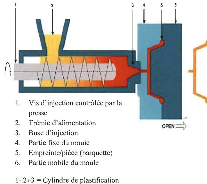
Figure 11 Schéma du procédé de moulage par injection
