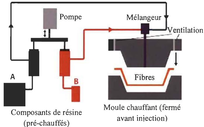
Figure 13 Schéma du procédé d'injection basse pression RTM
