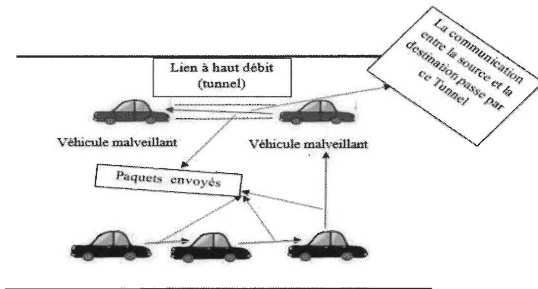
Figure 4 : L'attaque « Wormhole ».
