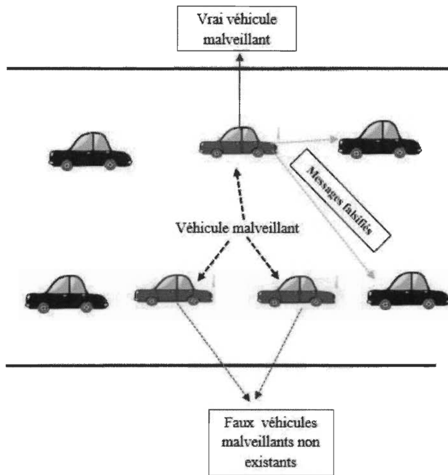
Figure 7 : L'attaque Sybil.
