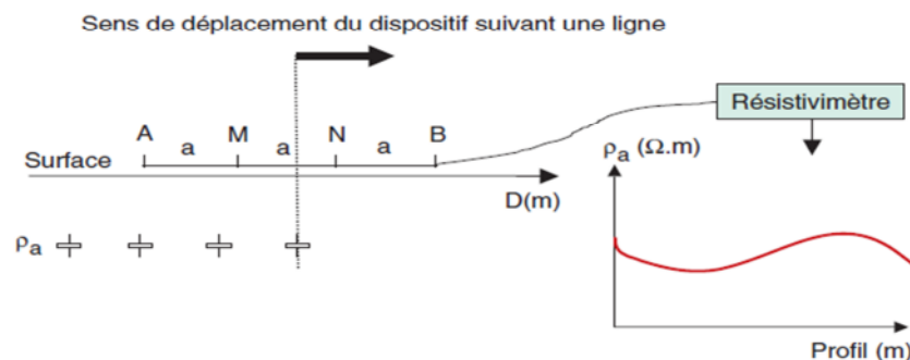
Figure 2.24 : Principe du traîné électrique, cas d'un dispositif Wenner.
