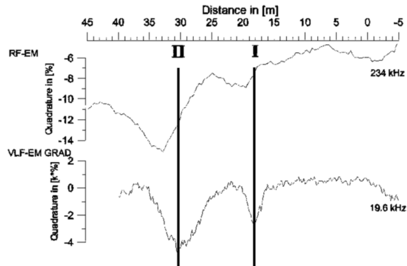
Figure 2.14: Comparaison entre les courbes enregistrées en continu par RF-EM et VLF-EM GRAD au passage de deux fractures dans des calcaires (Bosch, 2002).
