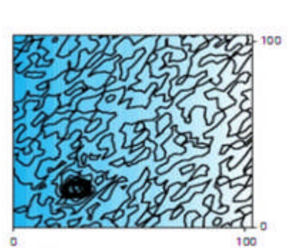
Figure 2.26c : anomalie résiduelle : différence entre l'anomalie de Bouguer et l'anomalie régionale.
