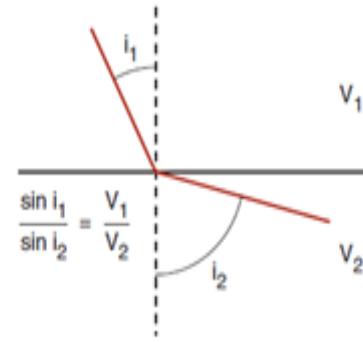
Figure 2.3 : Loi de Snell Descartes.
