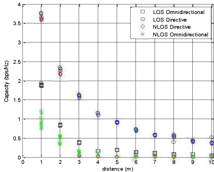
Figure 5-18: Capacité du canal au niveau 70m.
