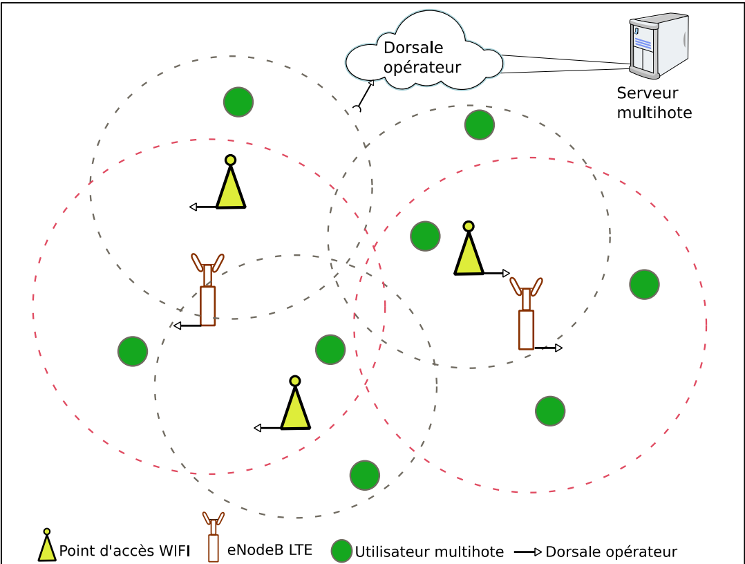
Figure 7.1 Vue schématique de la topologie pour la sélection des nœuds d'accès
