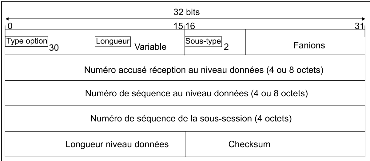
Figure-A I-4 Différents champs du sous-type Data Sequence Signal
