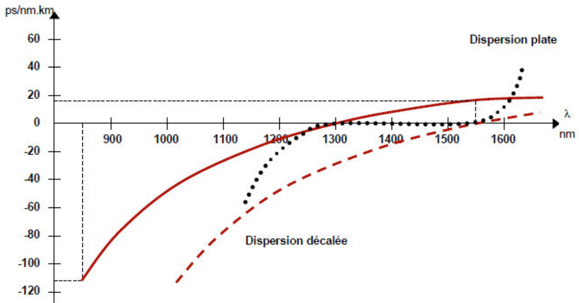
Figure 1.11 : Courbe de la dispersion chromatique.
