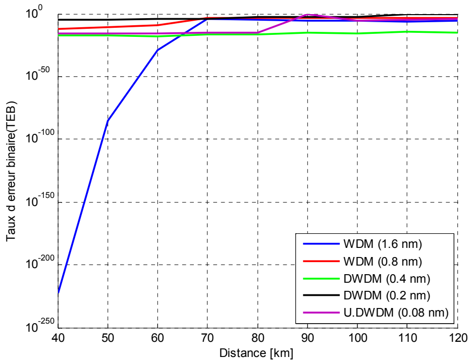
Figure 3.9 : Variation du taux d'erreur binaire en fonction de la distance.
