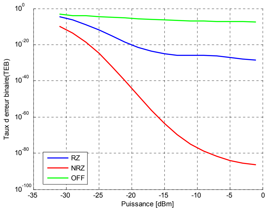
Figure 3.30 : Variation du taux d'erreur binaire en fonction de la puissance.
