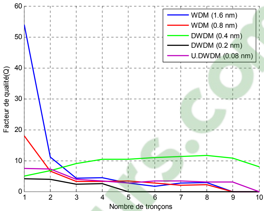
Figure 3.10 : Variation du facteur de qualité en fonction du nombre de tronçons.
