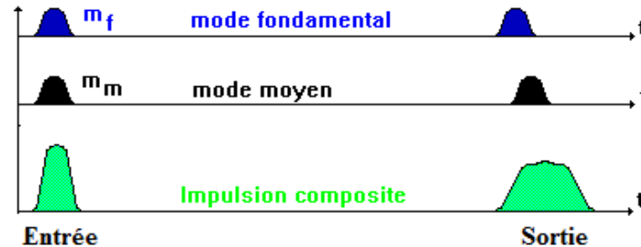
Figure 1.10 : Retard des modes.
