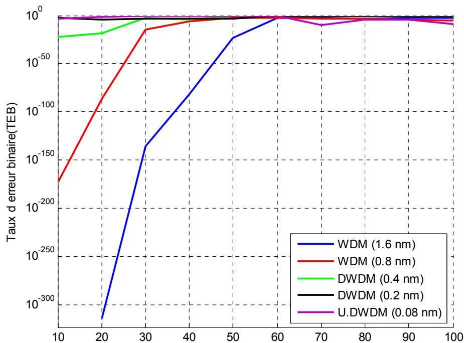
Figure 3.13 : Variation du taux d'erreur binaire en fonction du débit.
