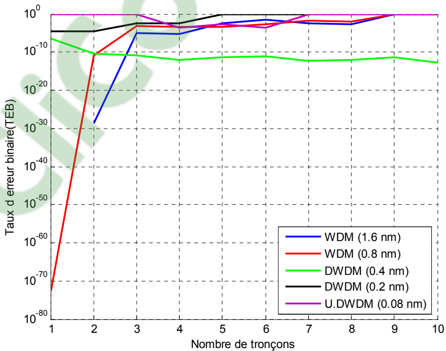
Figure 3.11 : Variation du taux d'erreur binaire en fonction du nombre de tronçons.
