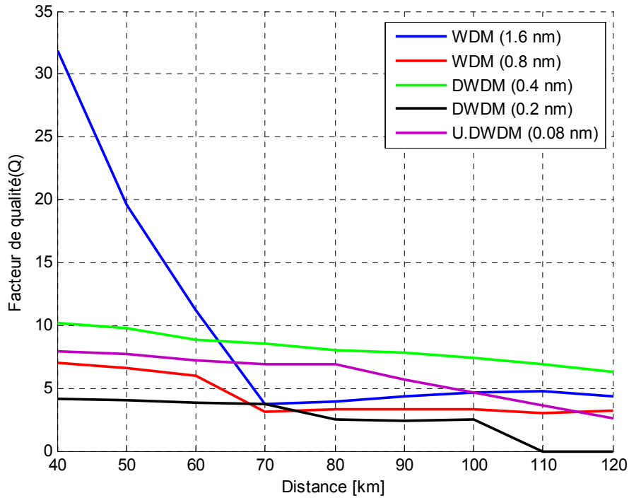
Figure 3.8 : Variation du facteur de qualité en fonction de la distance.
