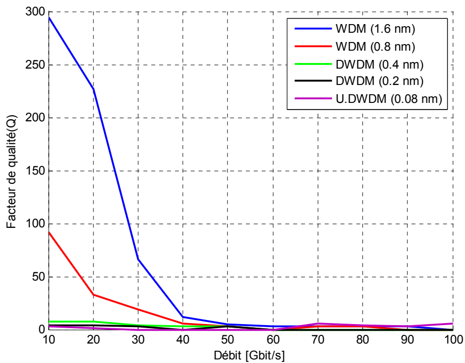
Figure 3.18 : Variation du facteur de qualité en fonction du débit.
