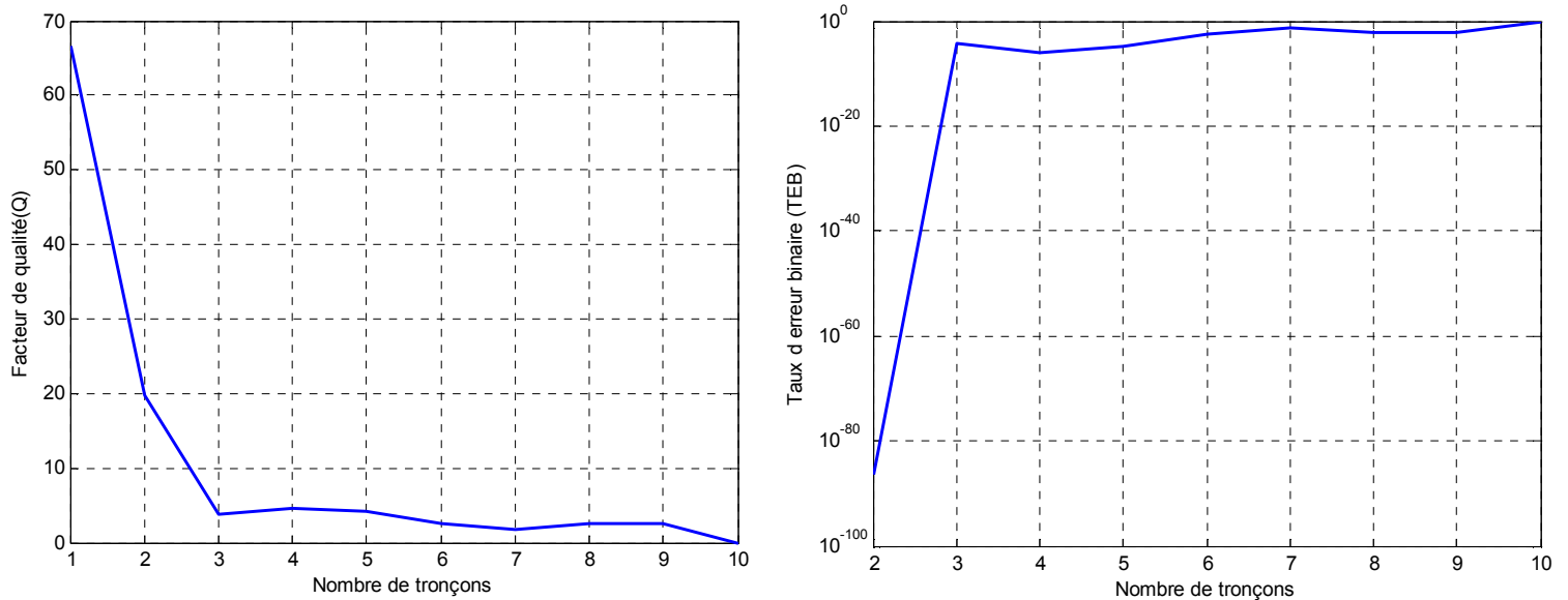
Figure 3.24 : Variation du facteur de qualité et du taux d'erreur binaire en fonction de nombre de tronçons.
