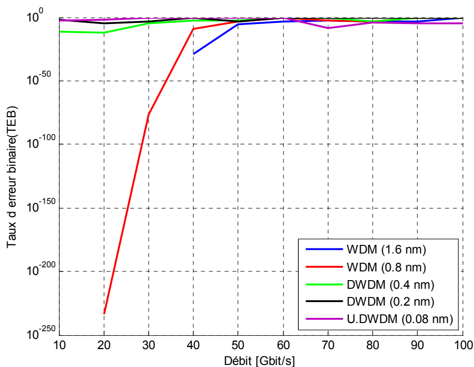
Figure 3.7 : Variation du taux d'erreur binaire en fonction du débit.
