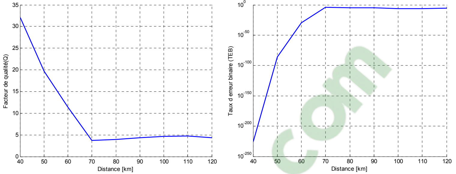
Figure 3.25 : Variation du facteur de qualité et du taux d'erreur binaire en fonction de la distance.
