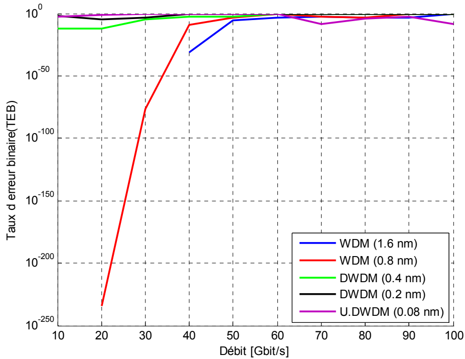
Figure 3.19 : Variation du taux d'erreur binaire en fonction du débit.
