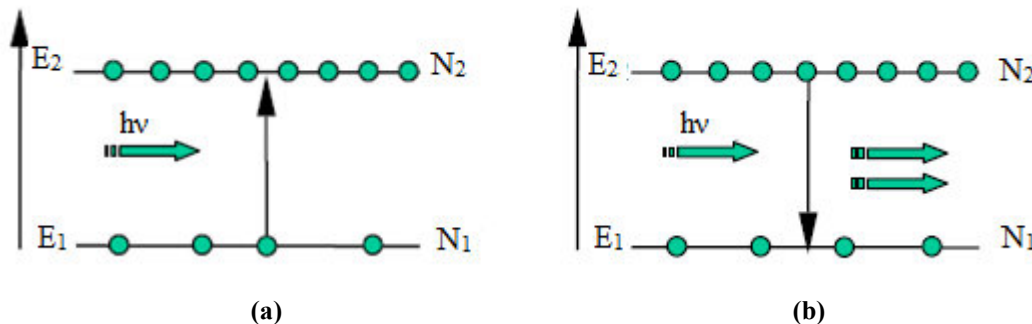
Figure 1.13 : Schéma des processus d'absorption (a) et de l'émission stimulée (b).
