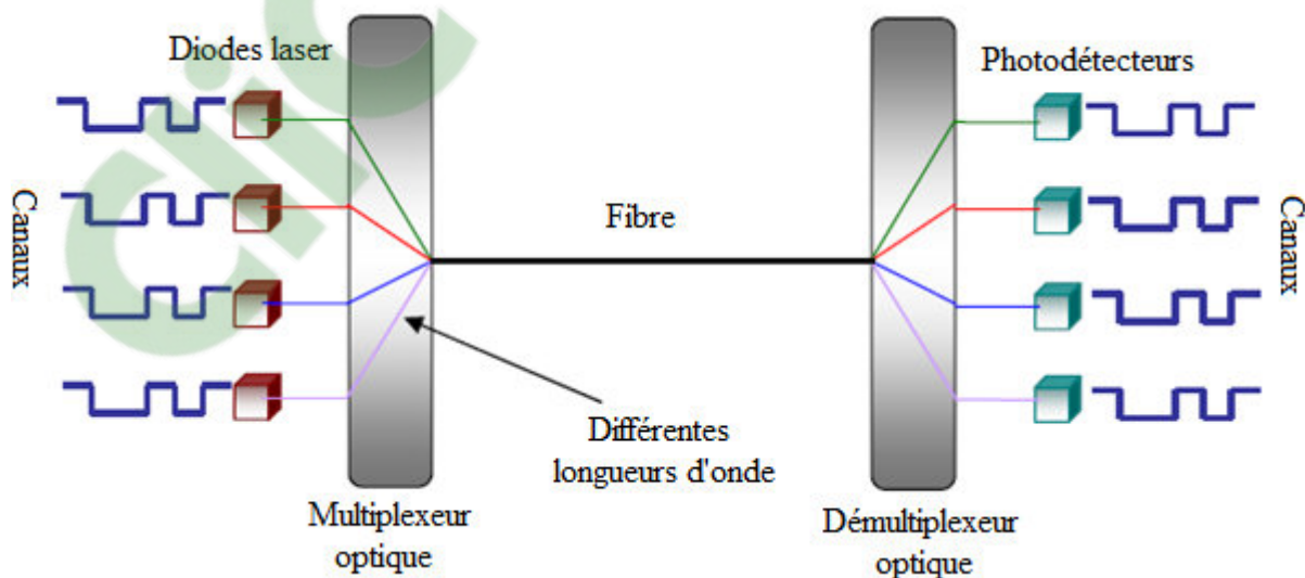
Figure 2.3 : Schéma de principe du multiplexage en longueur d'onde.
