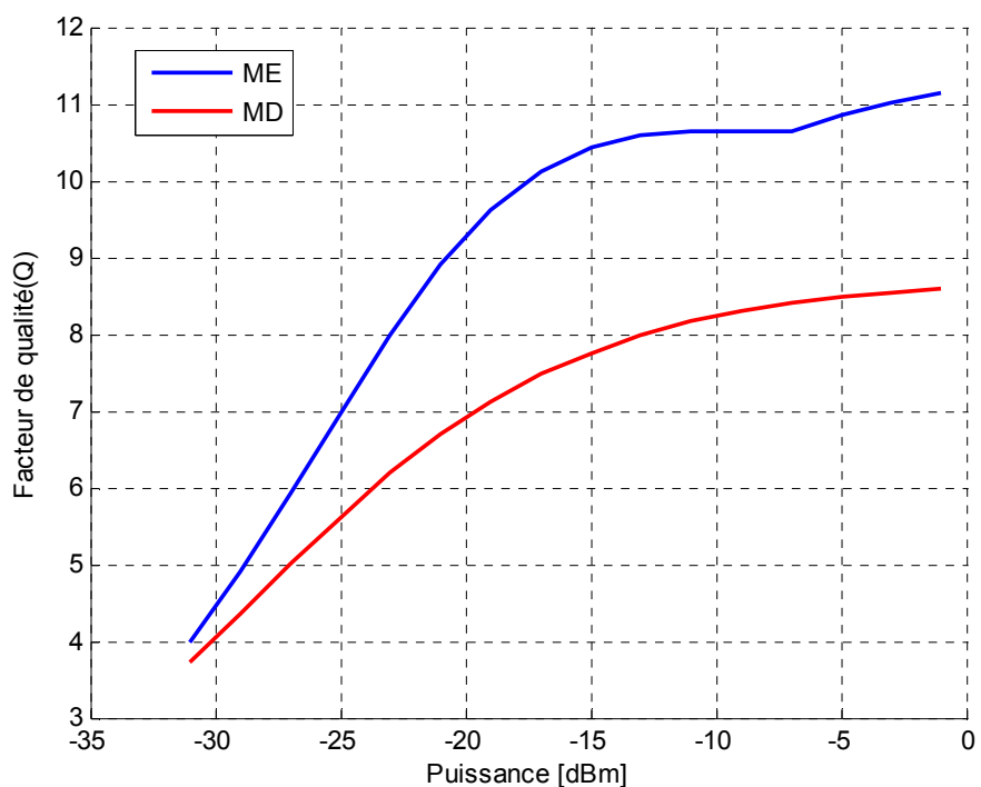
Figure 3.33 : Variation du facteur de qualité en fonction de la puissance.
