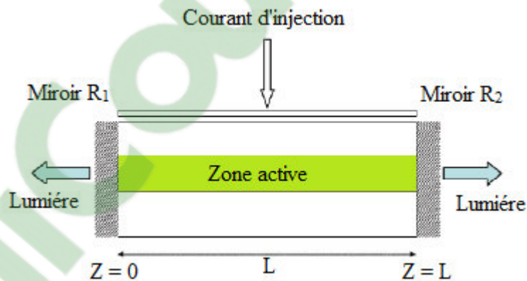
Figure 1.15 : Structure d'une diode laser à une cavité résonante Fabry-Perot.
