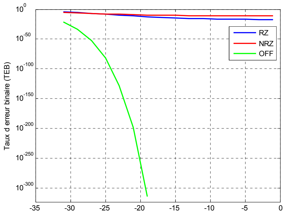
Figure 3.32 : Variation du taux d'erreur binaire en fonction de la puissance.
