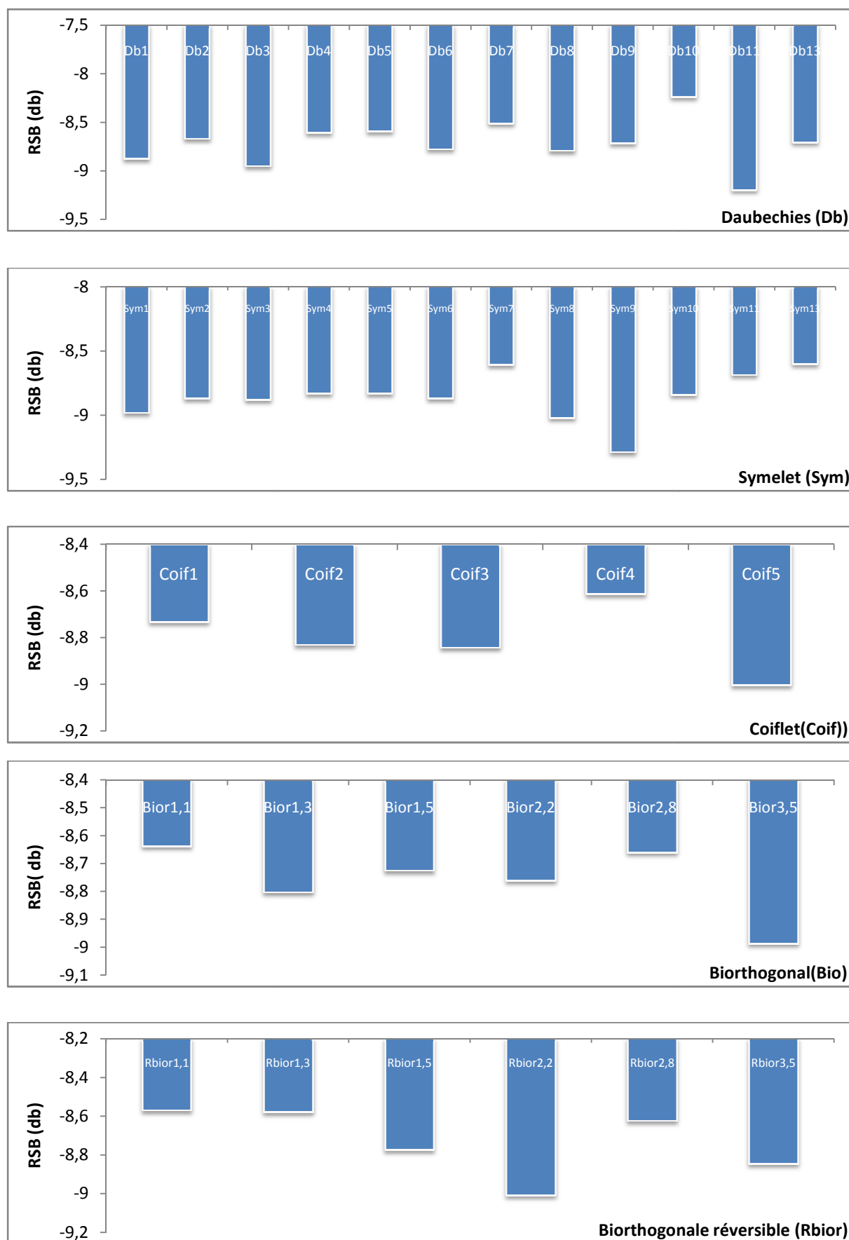
FIGURE 3.7. Choix d'ondelette par l'ajout de bruit d'un degré de bruit =3
