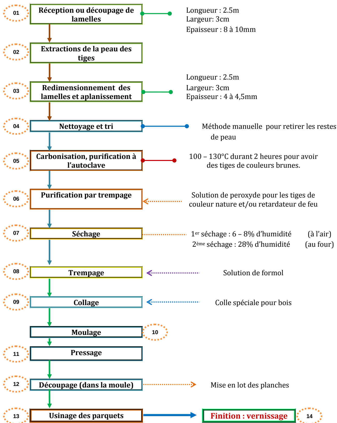
Figure n° 7 : Schéma de procédé de fabrication de parquet et de plancher de bambou
