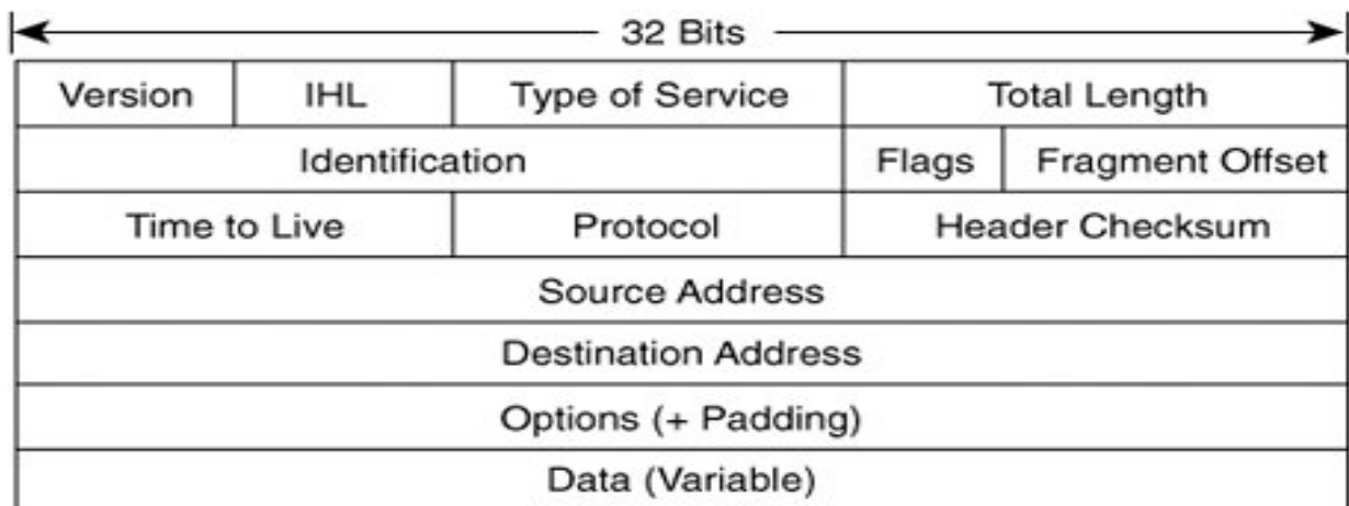
Figure 1.4 : l'entête IP version 4
