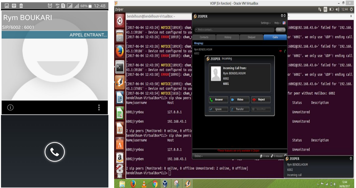
Figure 2.15 : Appel entrant du serveur vers notre client
