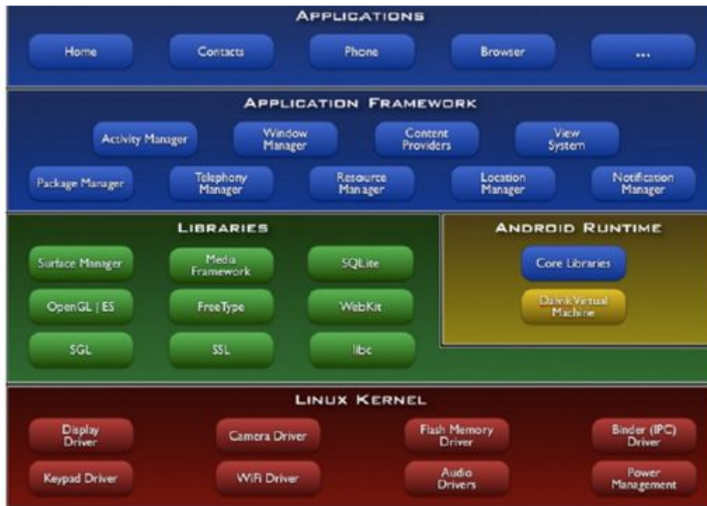
Figure 2.9 : Le noyau Android
