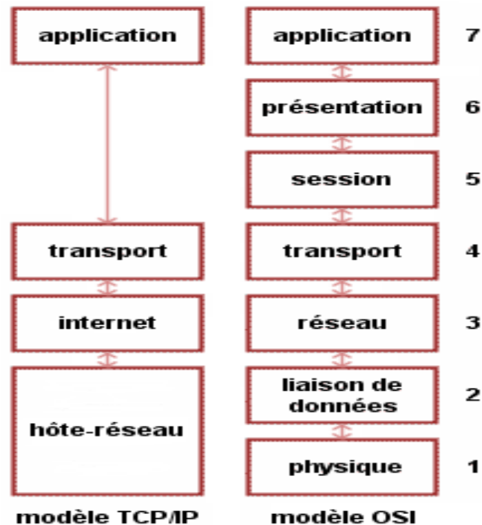
Figure 1.6 : Le modèle TCP vs OSI
