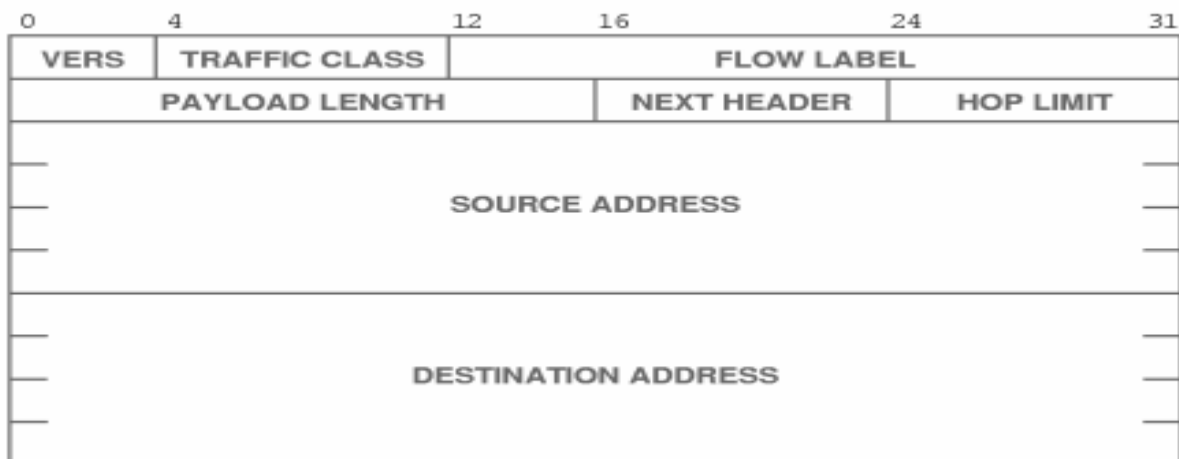
Figure 1.5 : l'en-tête IP version 6
