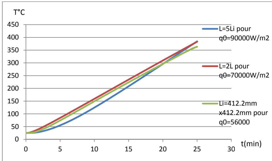
Figure 4.16 Comparaison des cycles de chauffage de la pièce en forme T pour les 3 largeurs de la pièce
