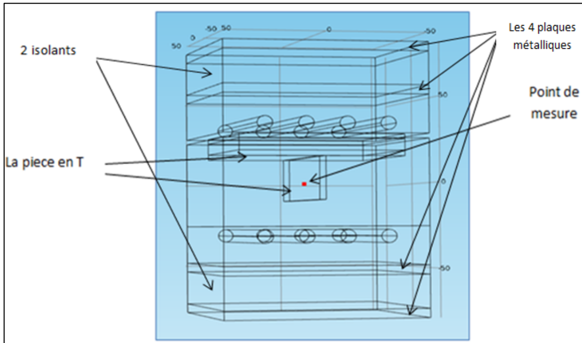
Figure 2.18 Le modèle de chauffage de la pièce en forme T
