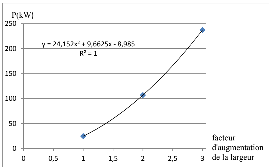
Figure 4.35 L'effet de la largeur sur la puissance de chauffage de la pièce concave
