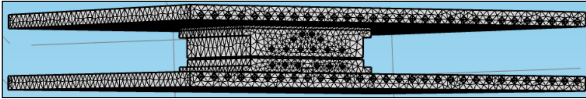
Figure 2.29 Le maillage la pièce concave dans le moule
