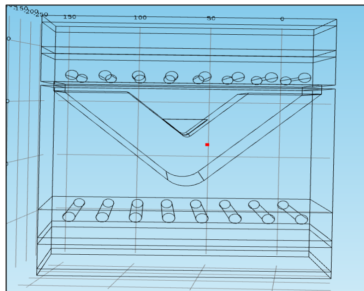
Figure 2.32 Le modèle de chauffage de la pièce en forme L 6 fois plus épaisse
