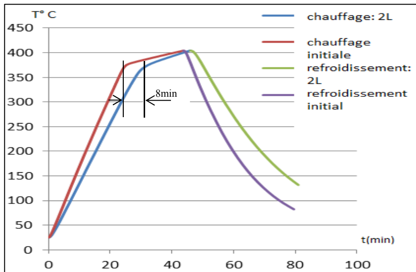
Figure 3.14 L'effet de 2 fois la largeur de la pièce sur le cycle de chauffage et de refroidissement
