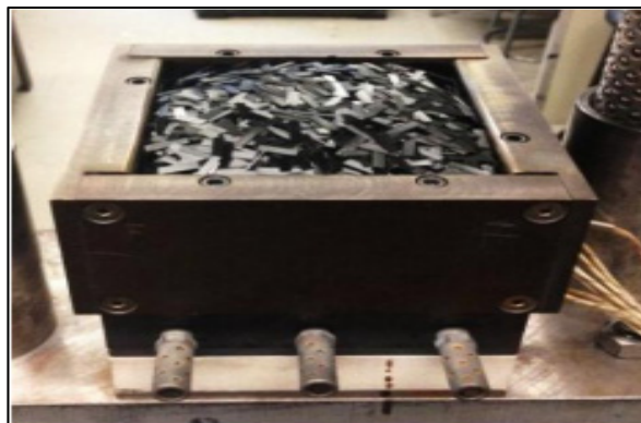
Figure 1.2 La cavité de la pièce en forme T remplie de brins tirés de Wazziki (2015, p.2)
