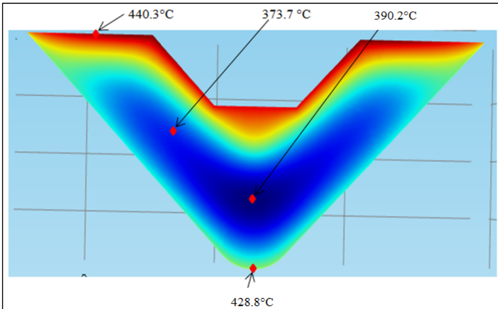
Figure 4.20 La répartition de la température dans la pièce en forme L après 30min de chauffage pour 6 fois l'épaisseur de la pièce
