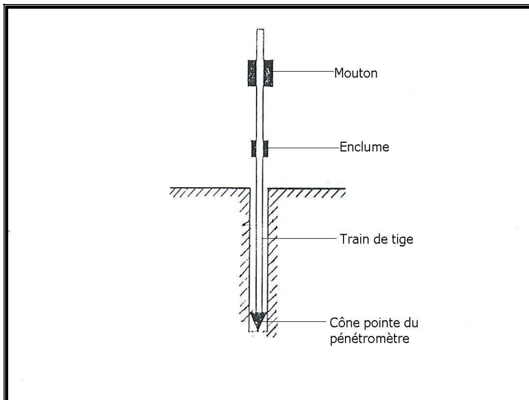
Figure 6: Pénétromètre dynamique
