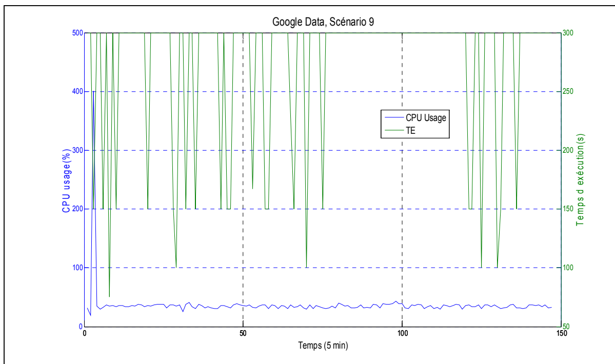
Figure 2.18 Scénario 9 - Variation des données réelles CPU et TE
