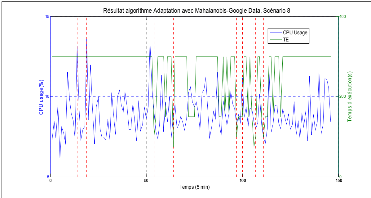
Figure IV.7 Scénario 8-Résultat de l'algorithme d'adaptation avec le Mahalanobis
