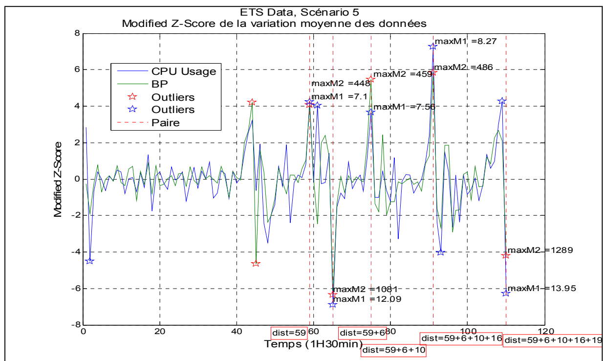
Figure 2.9 Scénario 5 - Valeur de Modified Z-score CPU et BP
