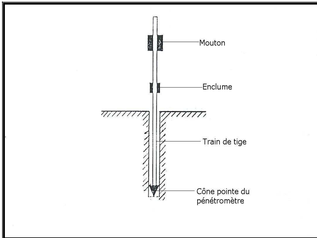
Figure 6: Pénétromètre dynamique
