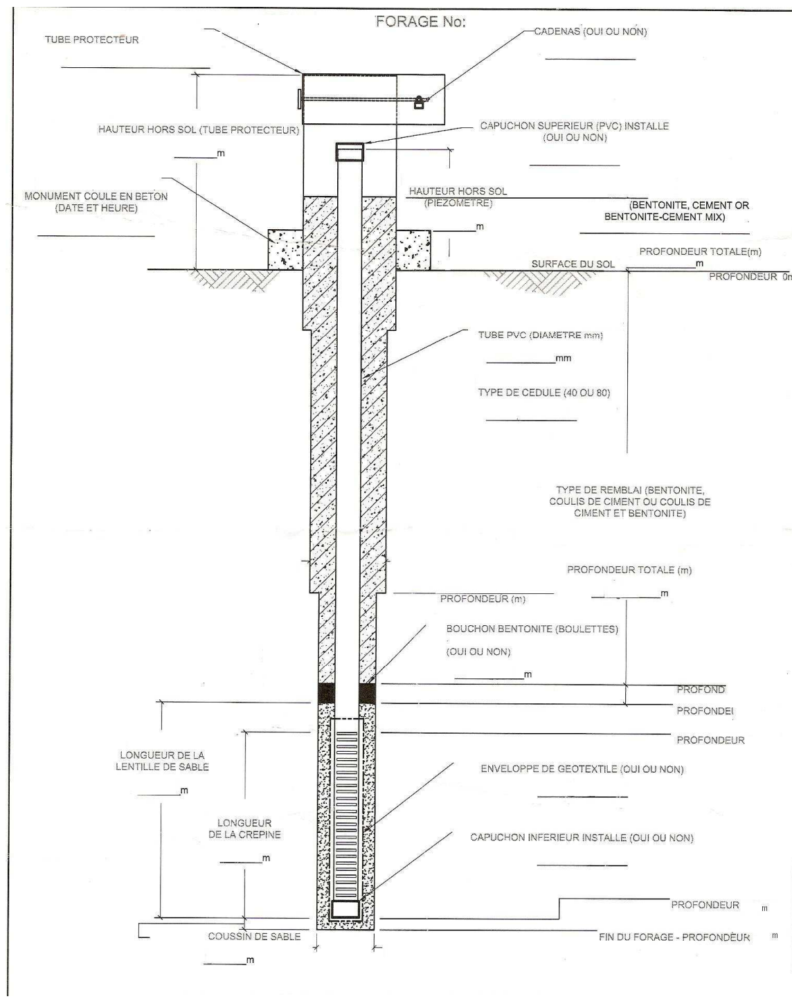
Figure 9: principe de piézomètre
