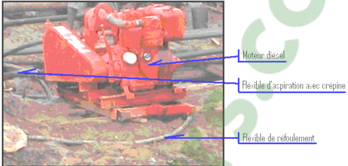
Photographie 2: Pompe à boue
