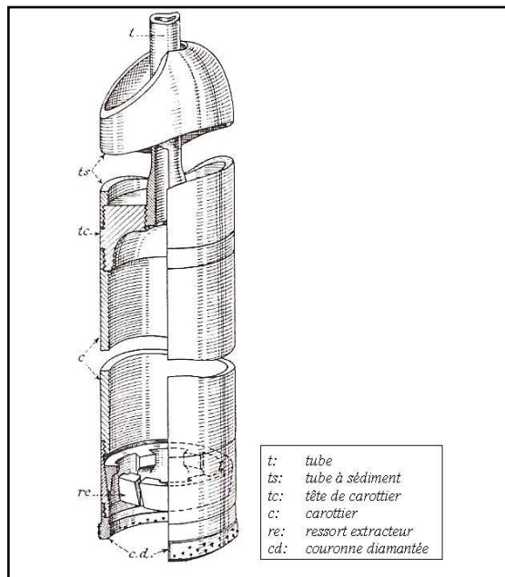
Figure 5: Tube carottier à couronne diamantée
