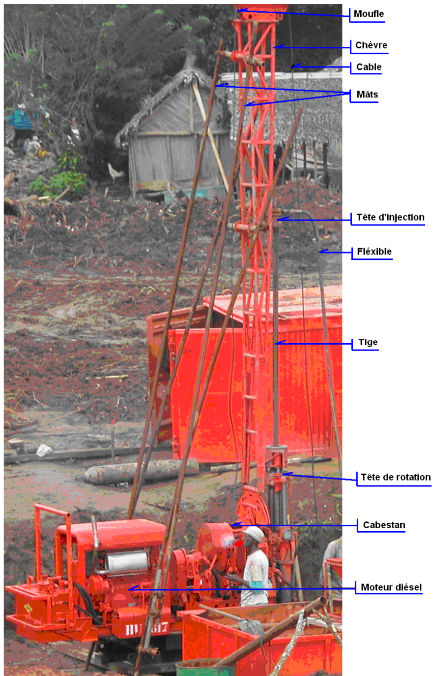
Photographie 1: Machine sondeur
