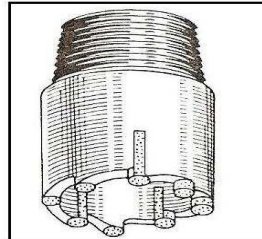
Figure 4: couronne à prismes de carbure de tungstène
