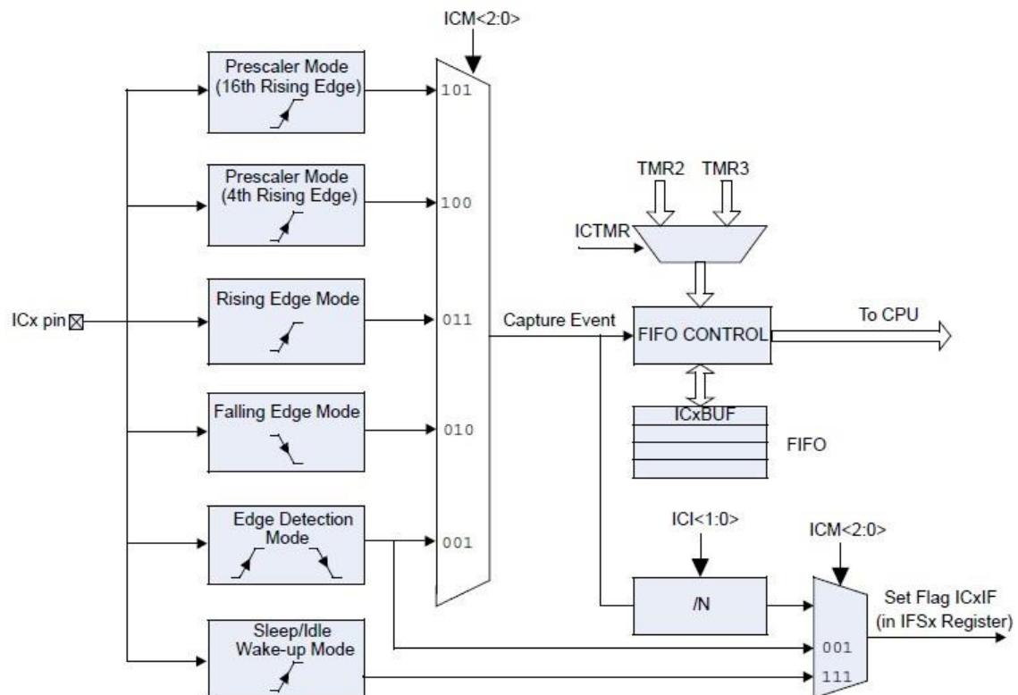
Fig4.10 : diagramme synoptique du circuit interne input capture
