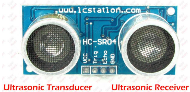
Figure4.5:vue de face de HC-SR04
